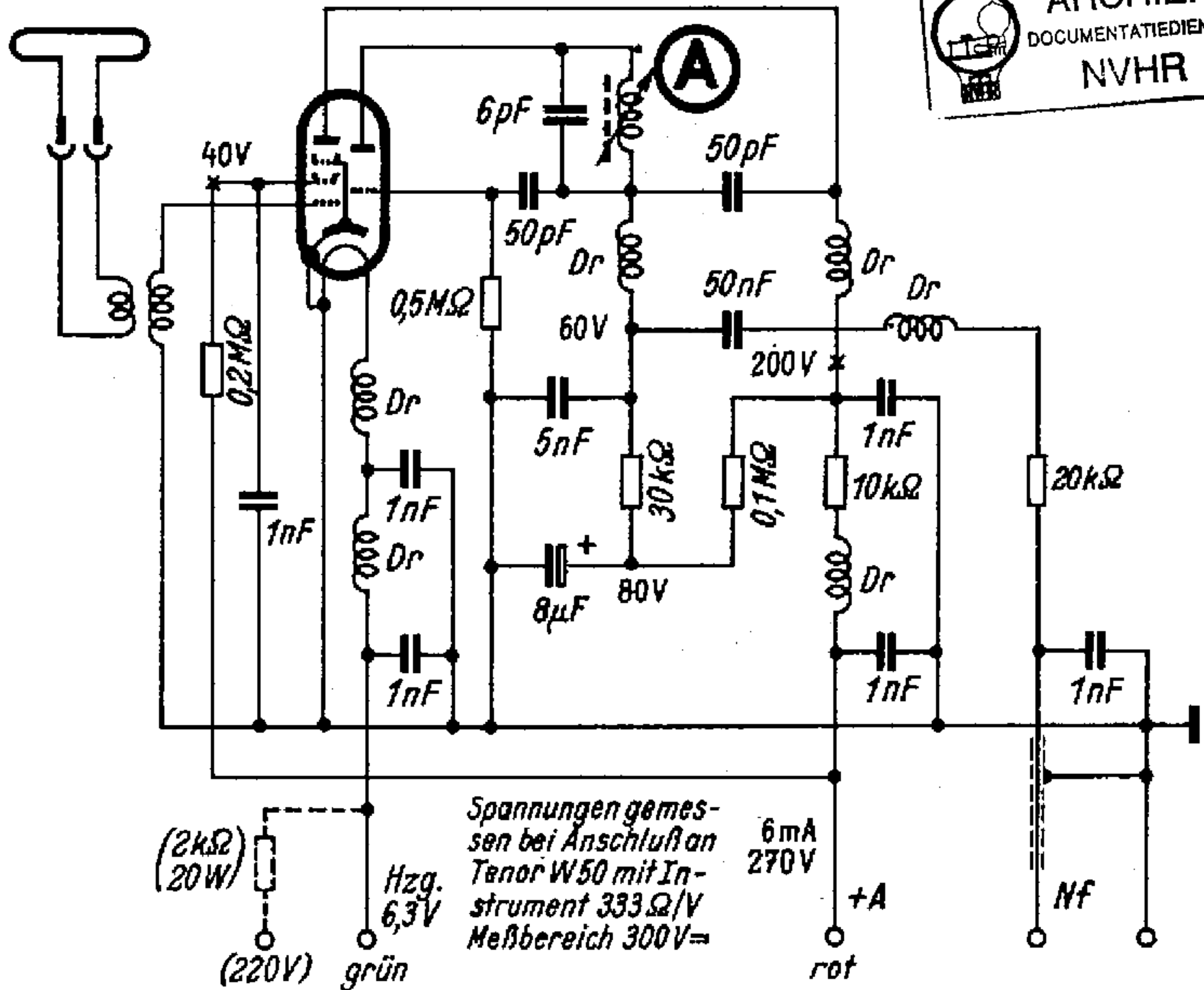
Kreff-UKW-Einbaugerät
