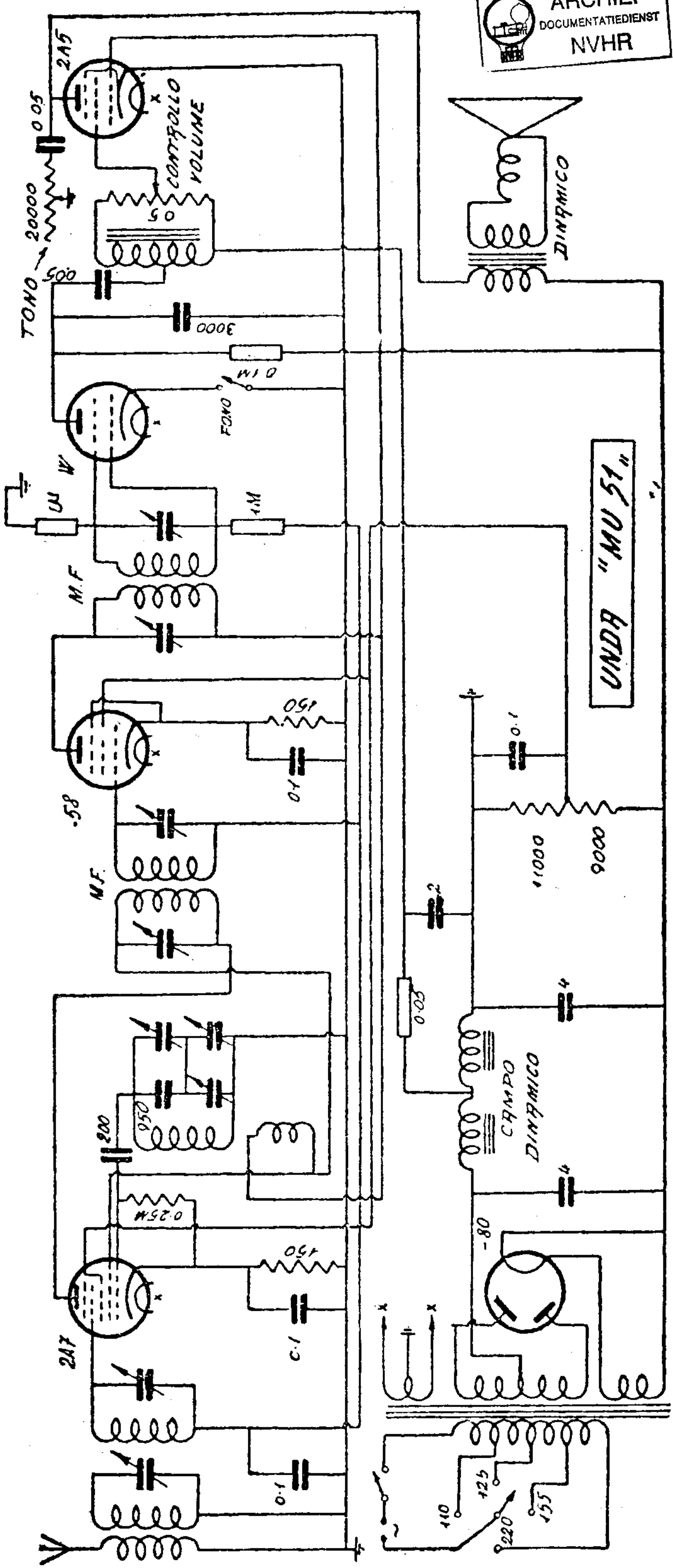
UNDA RADIO: — Modello « M. U. 51 ». - Produzione 1933. - Media frequenza: 175 kc.
