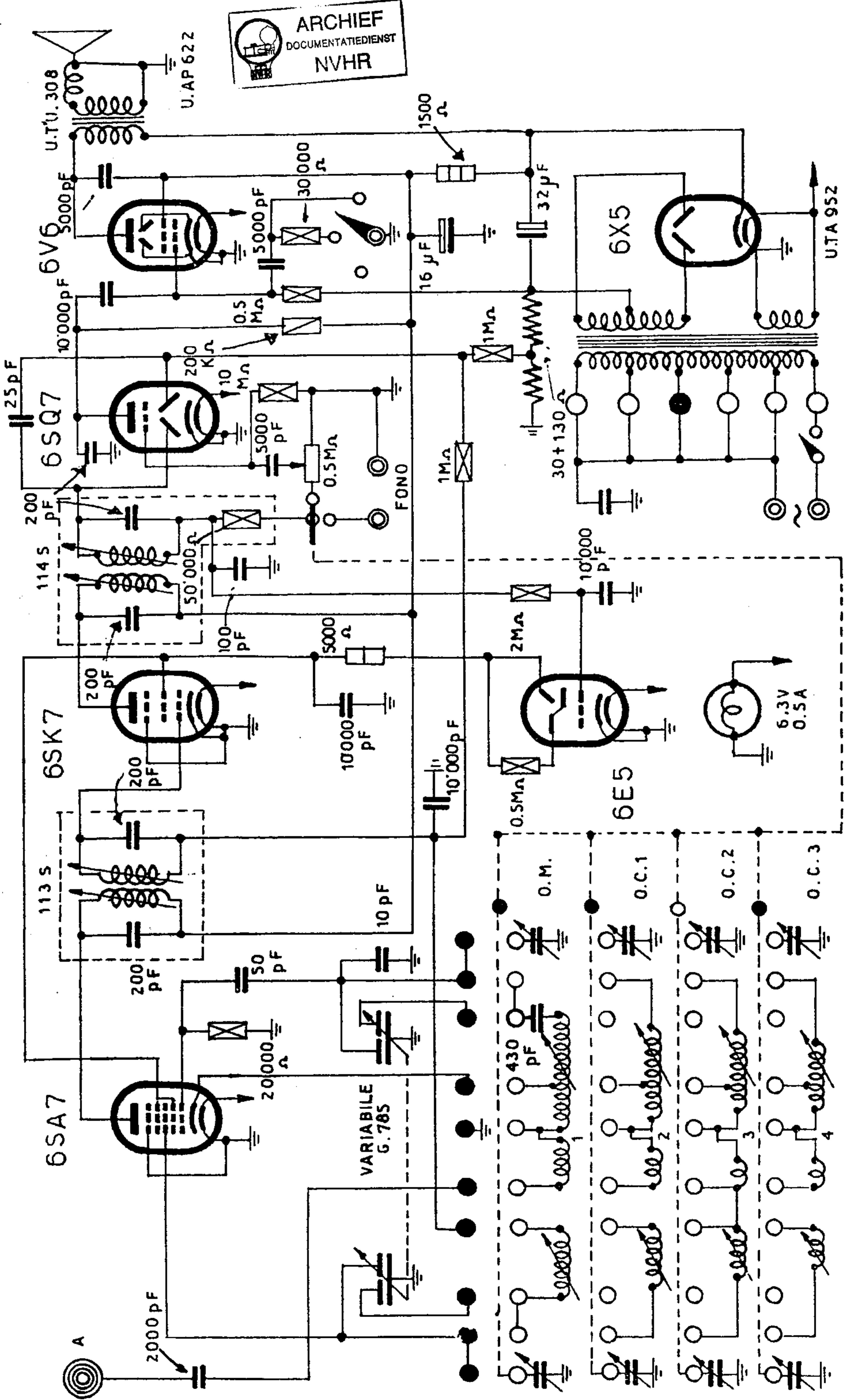
UNDA RADIO - Mod. R. 64/6 - Onde medie e tre corte. Gruppo AF a tamburo. Media frequenza a 450 kc. Finale placca 215 V schermo 180 V. Conv. e amplif. MF placca 180 V, schermo 110 V. Corrente anodica totale 50 mA.
