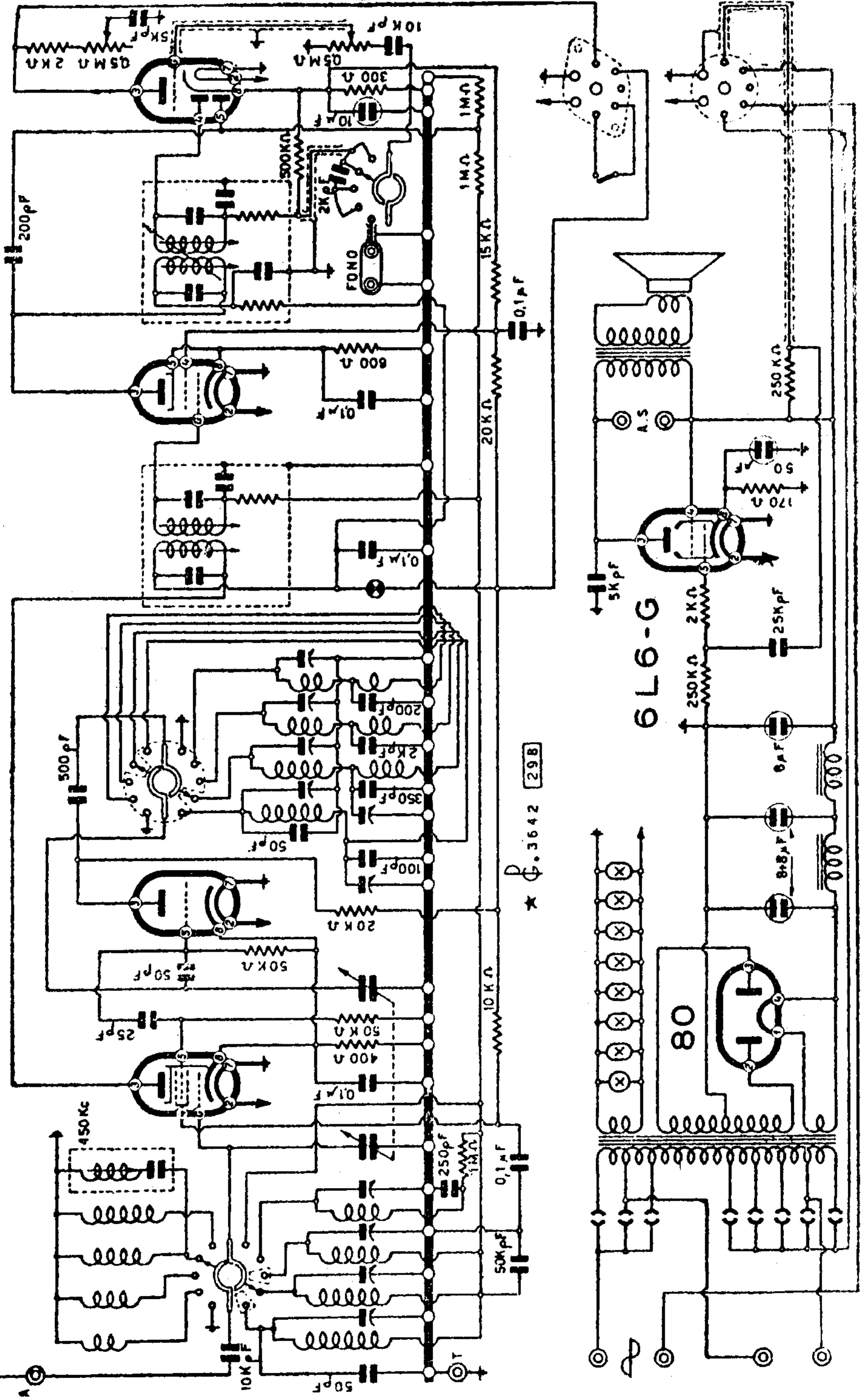
UNDA RADIO - MOD. « SUPER QUADRI UNDA 639 »
