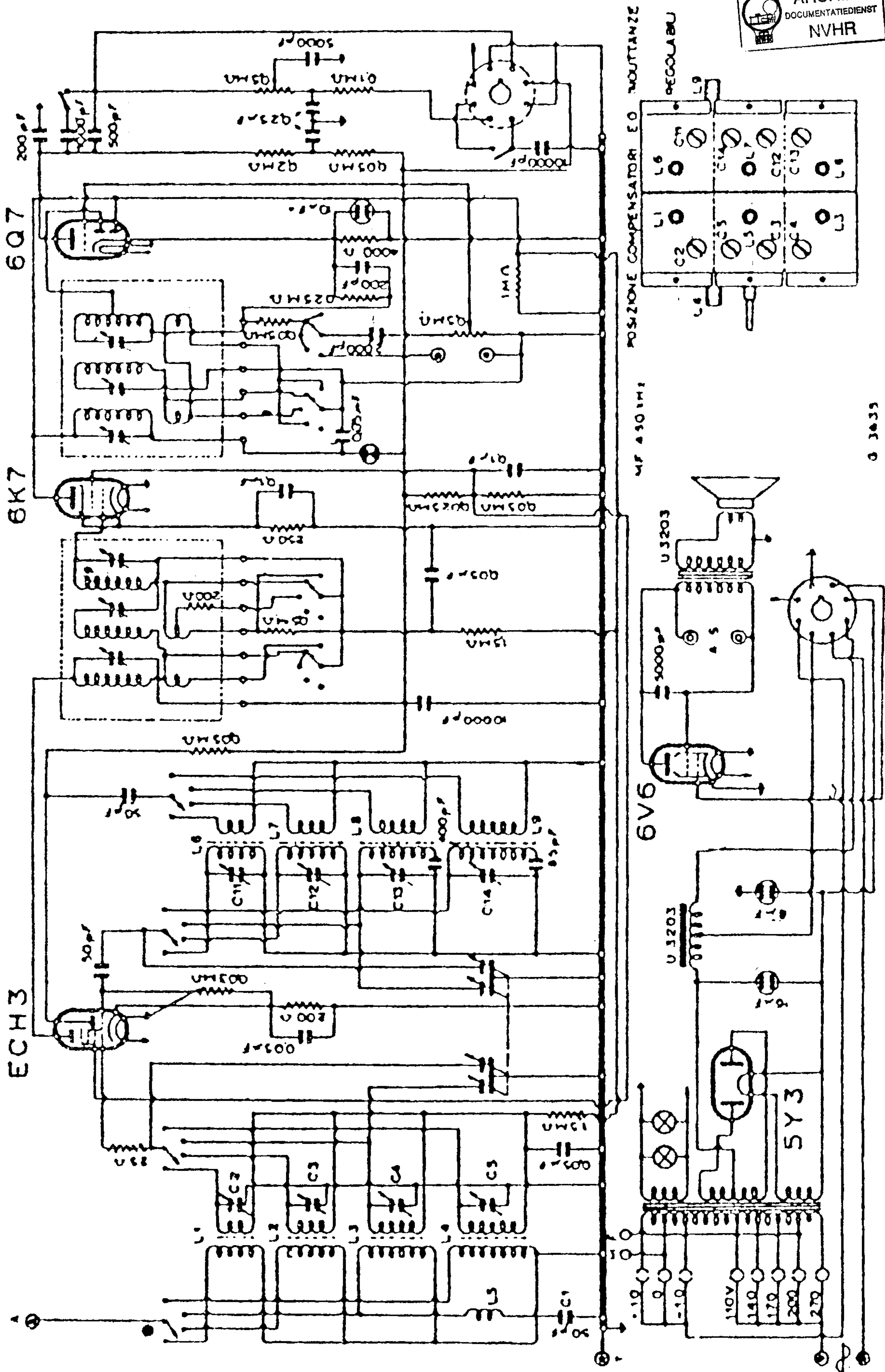
UNDA RADIO - MOD. « QUADRI UNDA 545 »
