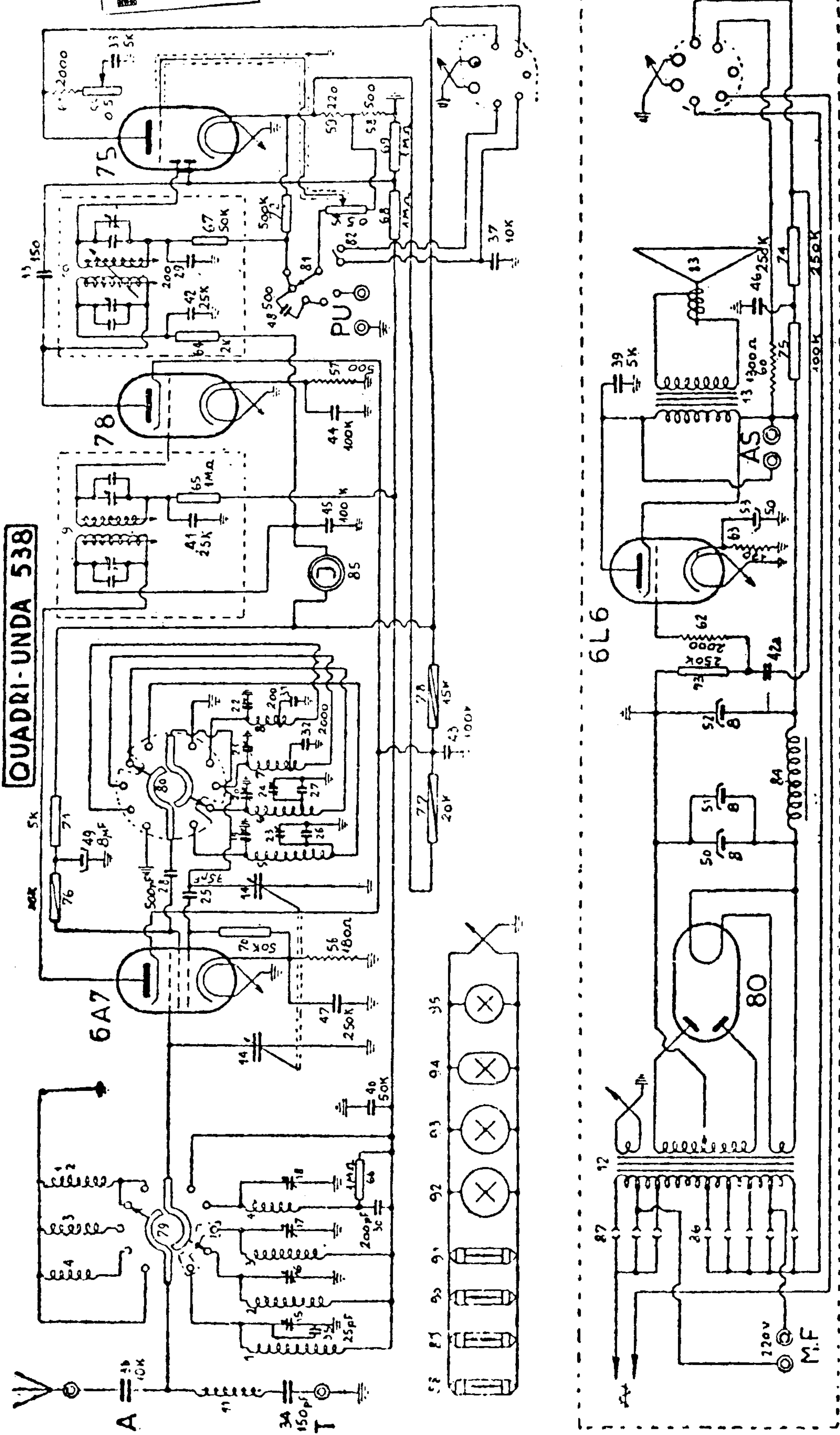
UNDA. RADIO. — Modello Super Quadri-Unda 538. — Produzione 1938-39. — Gamme: cc. (15,5-30), c. (30-80), m. (206,5-600), l. (750-2000). — Potenza d'uscita: 6.5 W. — Media frequenza: 450 kHz.
