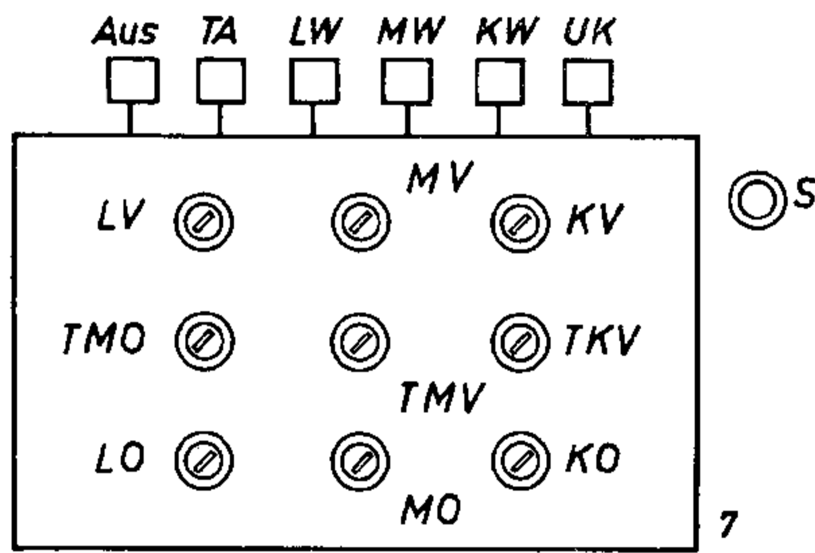
Spulensatz von unten
