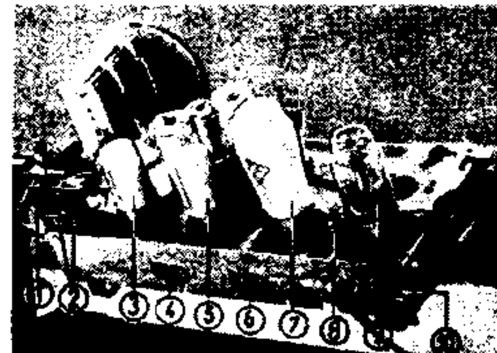
① Sperrkreis, ② Antennen- und Erdanschluß, ③ UCH 11, ④ Tonabnehmeranschluß, ⑤ UBF 11, ⑥ Anschluß für den zweiten Lautsprecher, ⑦ UCL 11, ⑧ Sicherung, ⑨ UY 11, ⑩ Tonabnehmereinschaltung
