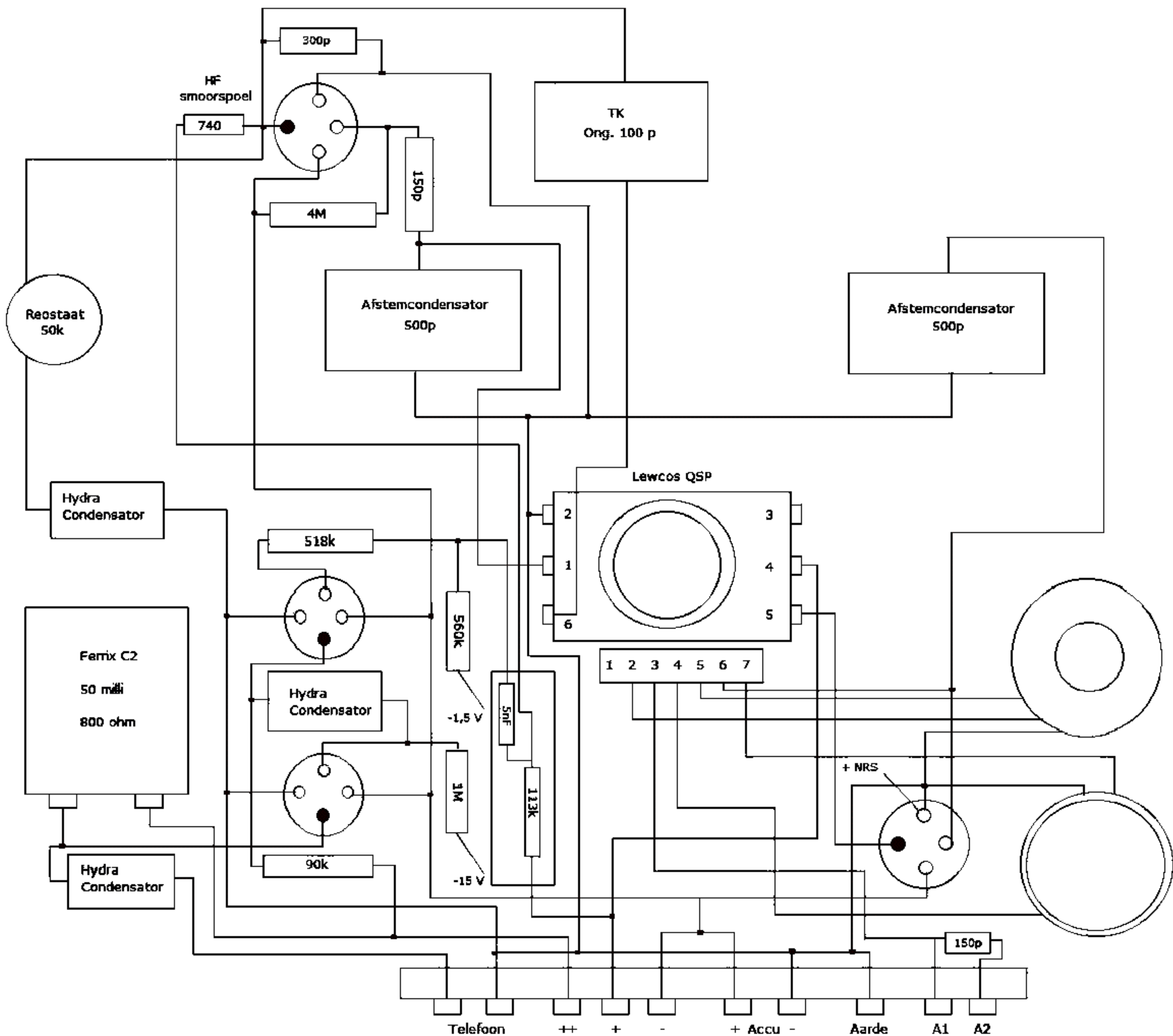
Bedradingschema Radio Tukker Sonora 4, 1927
