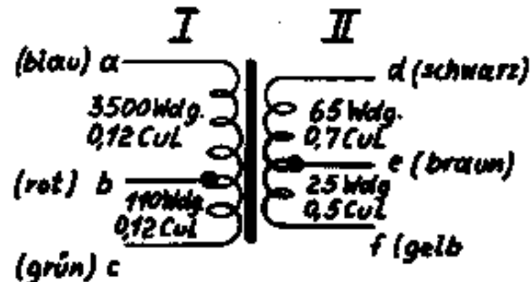
Wickeldaten für Ausgangs- übertrager 653-45/133-44
