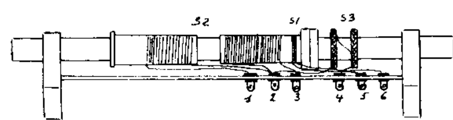
Cadre Ferrocube.
