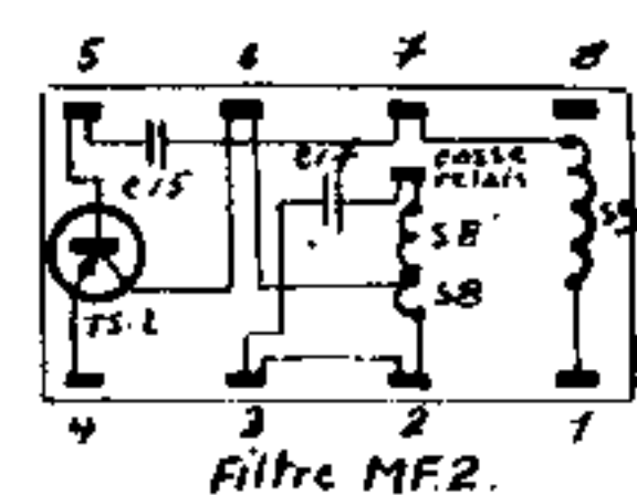
Filtre MF2.
