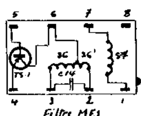
Filtre MF1.
