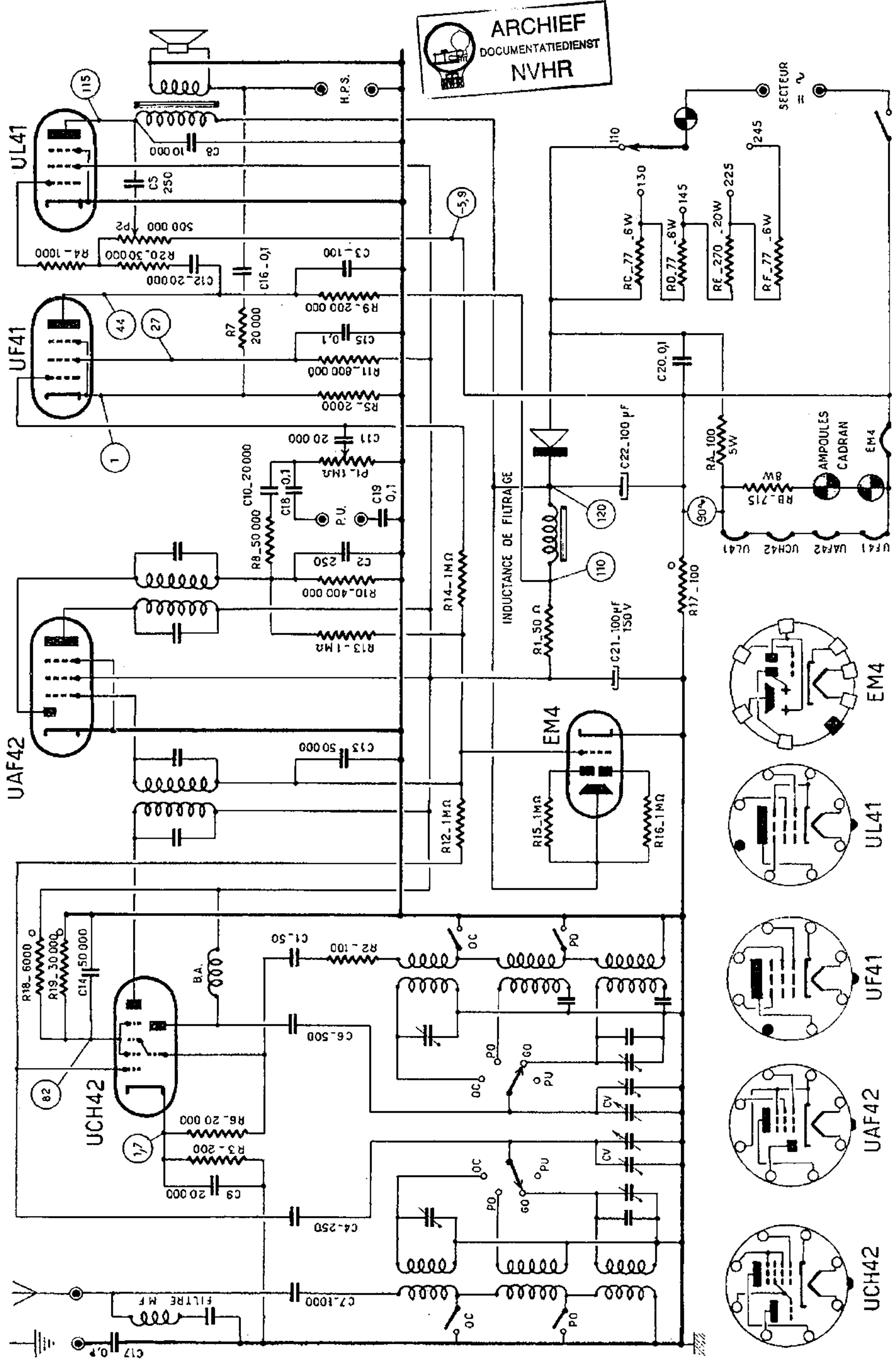
Schéma général des récepteurs Menuet 942TC et Duo 55TC dont la description se trouve page 82.
