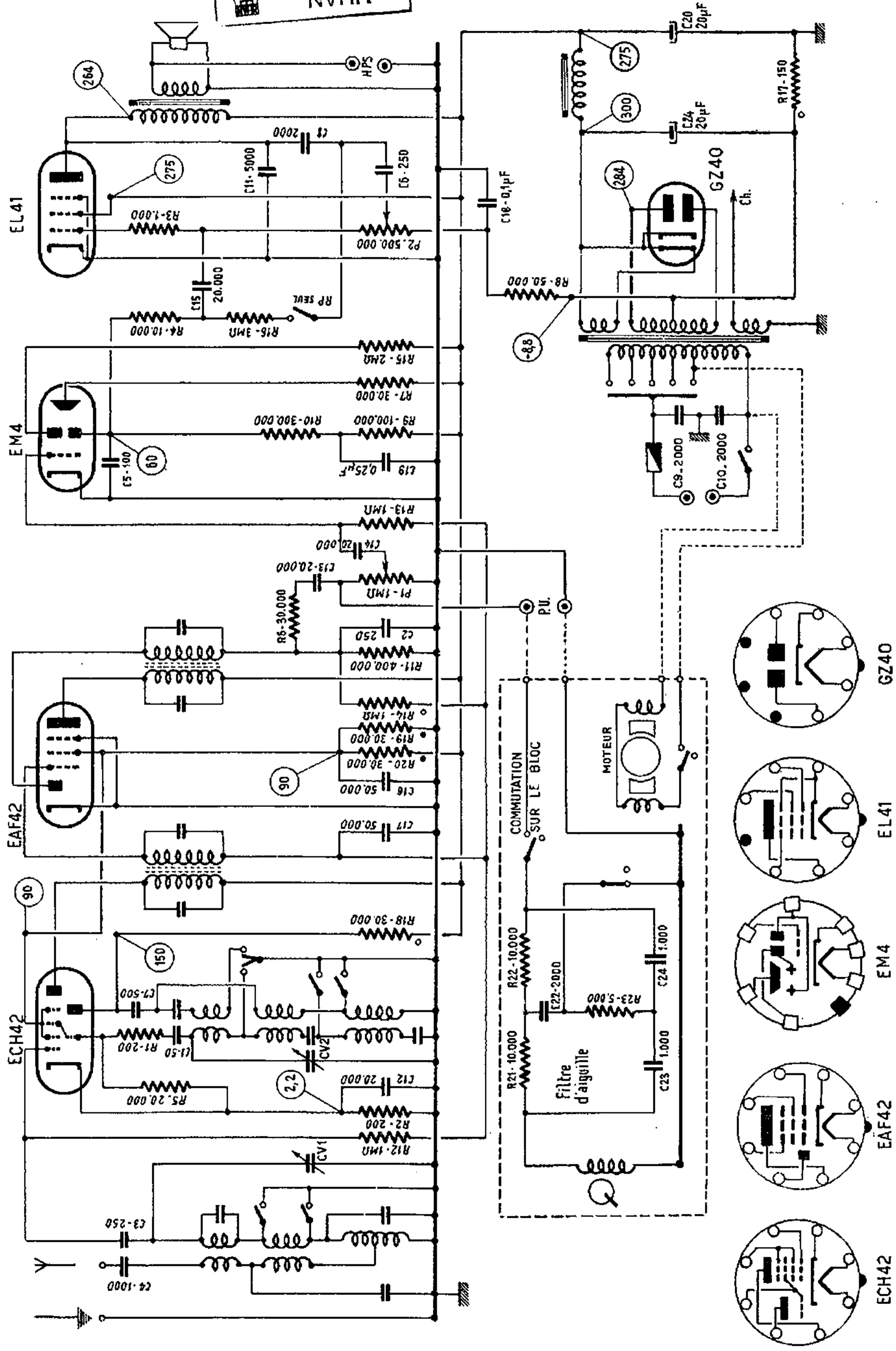
Schema général des récepteurs Menuet 942 et Menuet 53 dont la description se trouve page 82.
