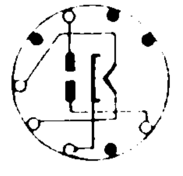
EZ80
