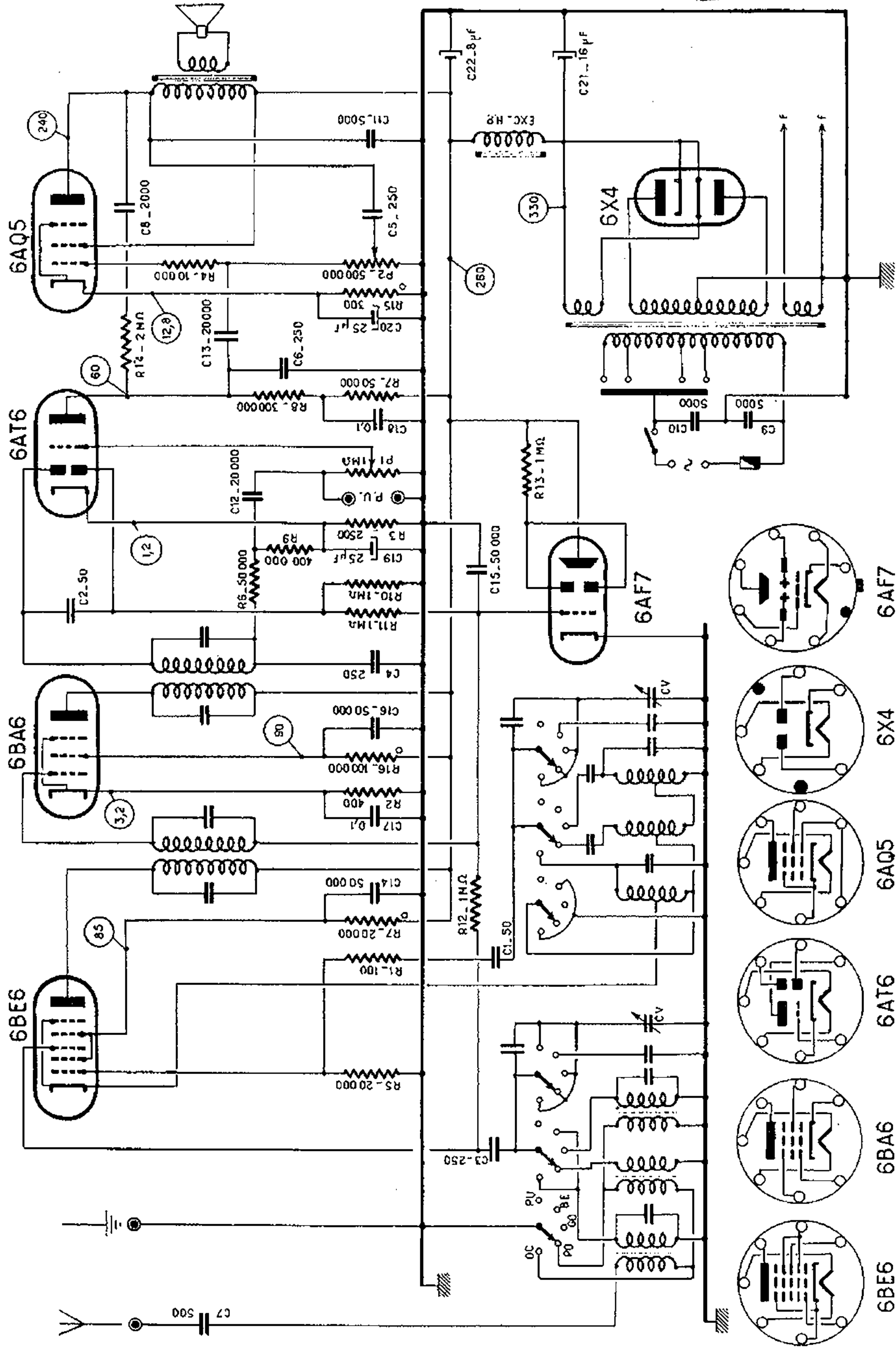
Schéma général du récepteur Airby 400, dont la description se trouve page 82.
