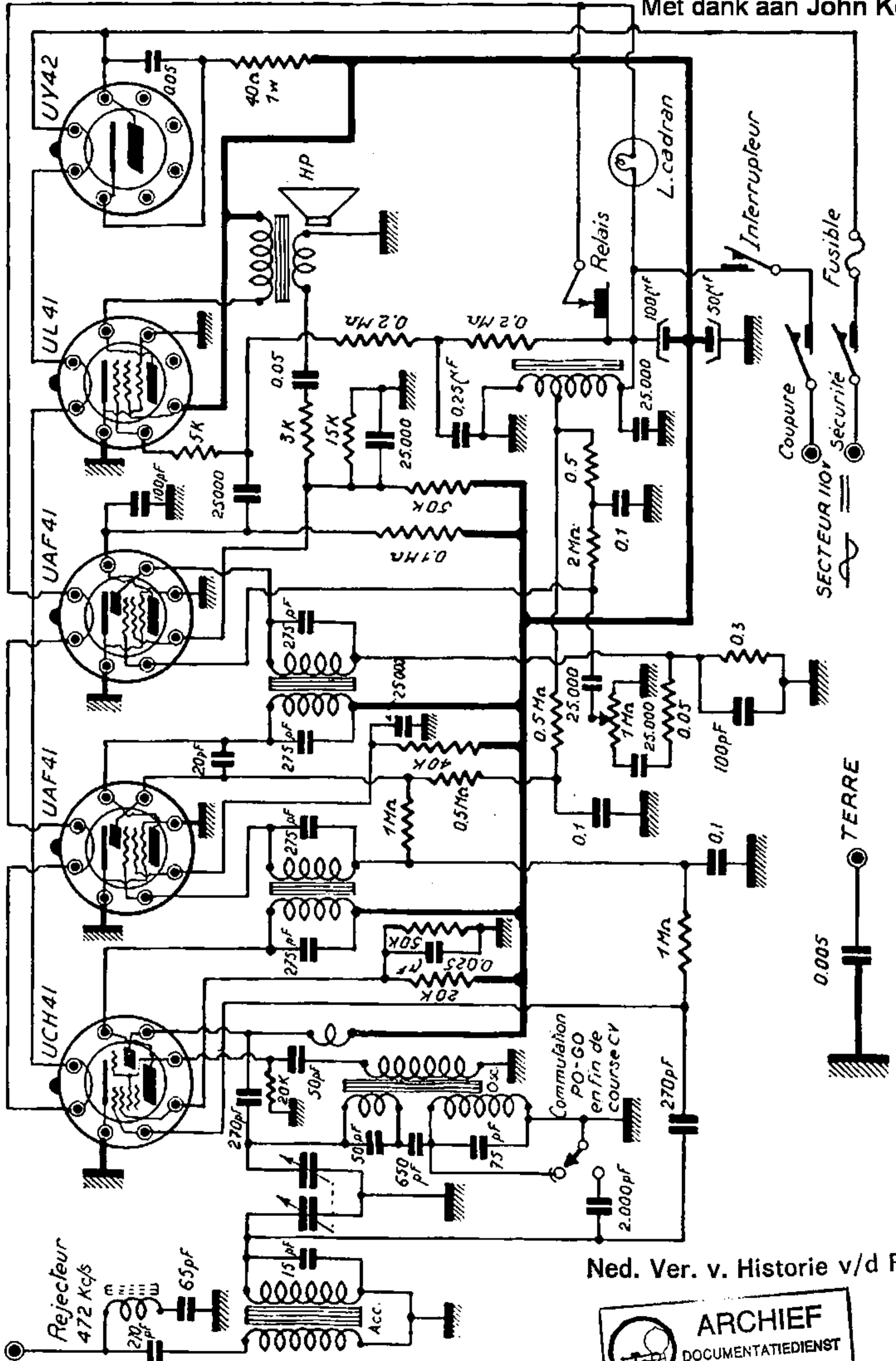
FIG. 2. — Schéma complet des circuits du Super-Bowm relevé sur le récepteur avec la collaboration des services techniques de Radiava. Ce schéma doit être aussi édité en notice de dépannage.
