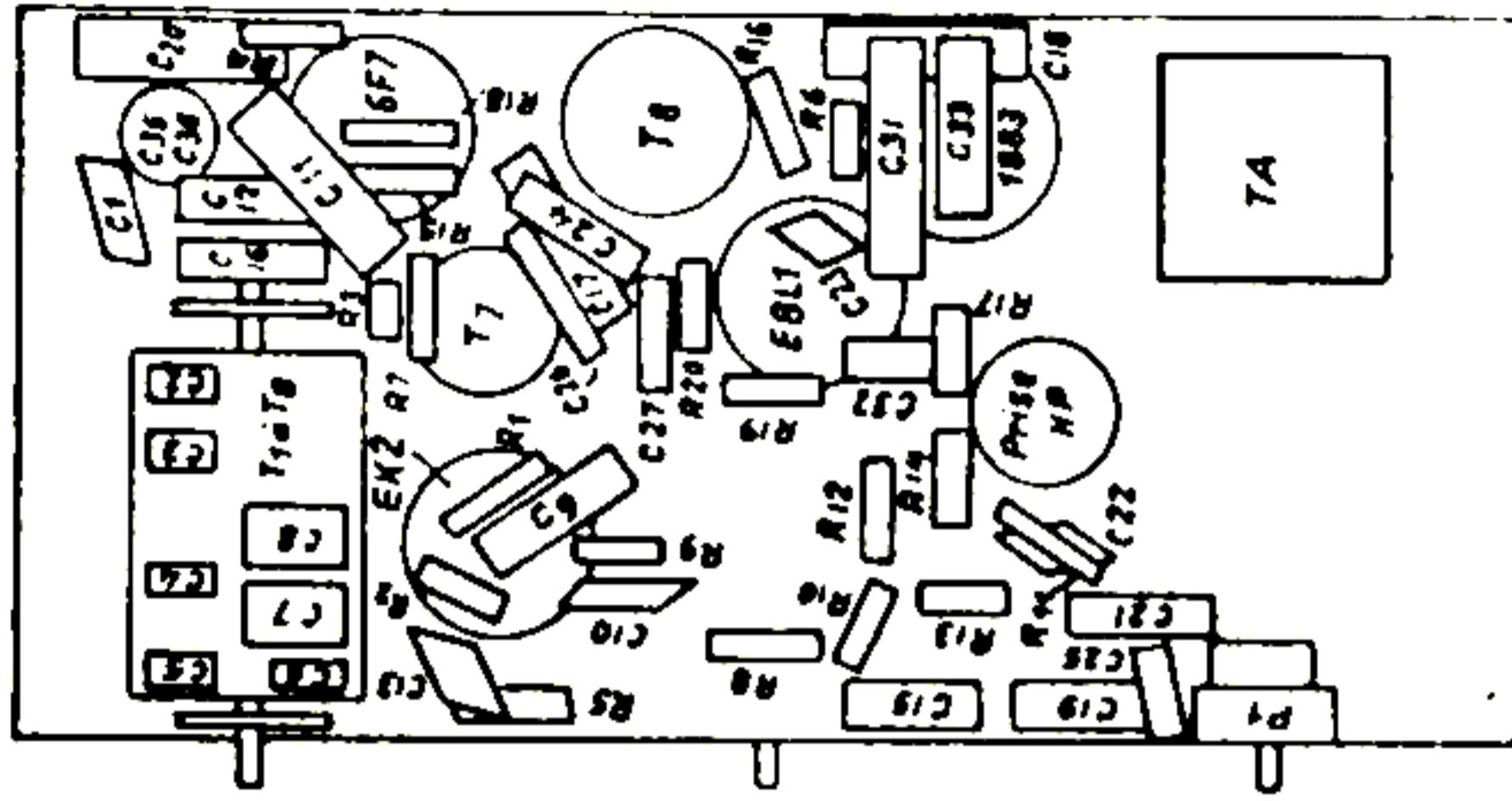
Disposition des éléments à l'intérieur du châssis M 49 — M 95.
