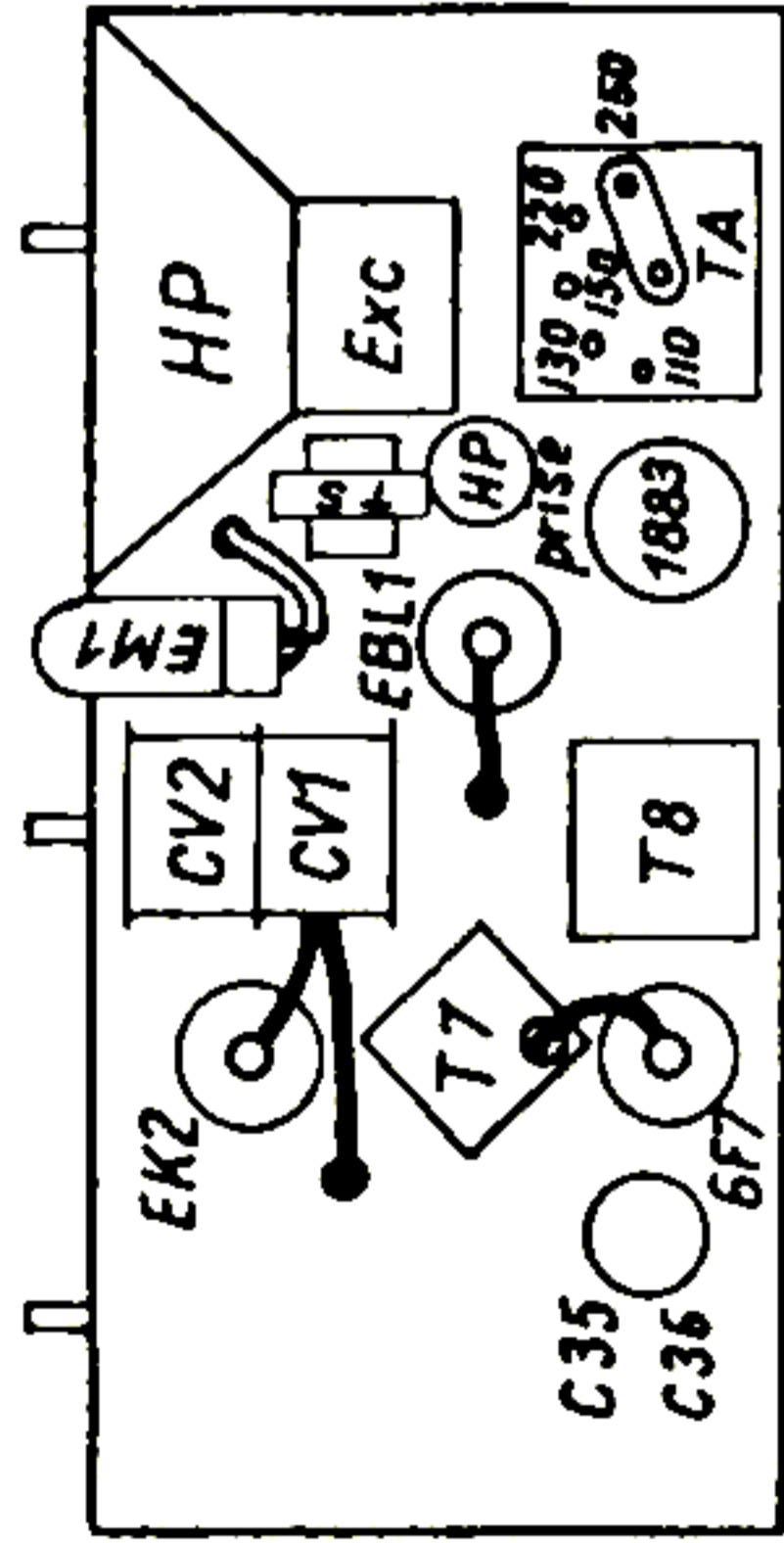
Disposition des éléments sur le dessus du châssis M 49 — M 95.
