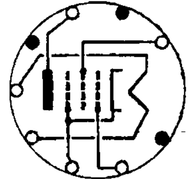
EL84
