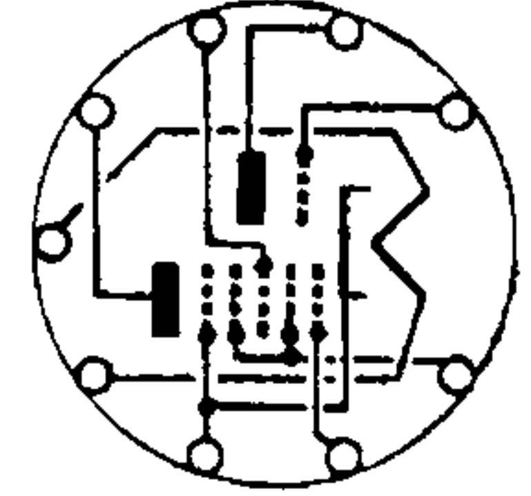
ECH81
