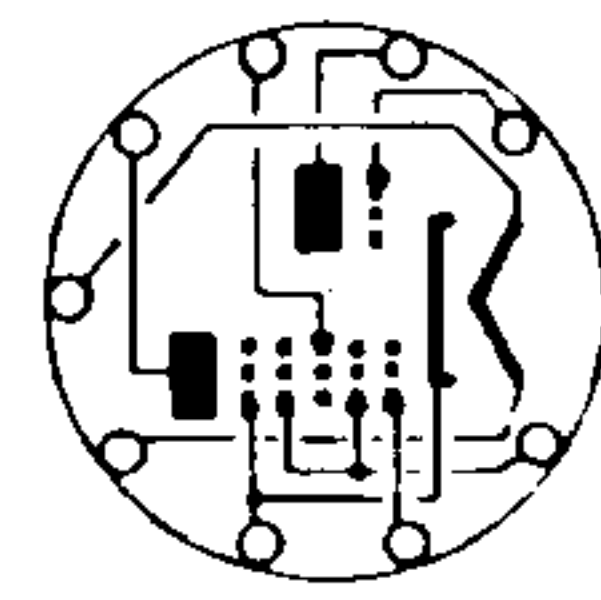
ECH81
