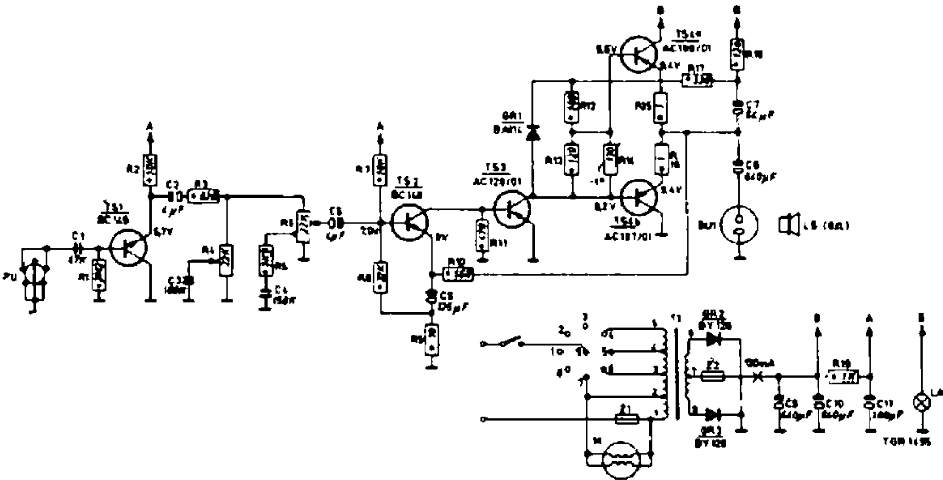
Fig. 70 – Amplificatore della fonovaligia Philips mod. 22GF632
