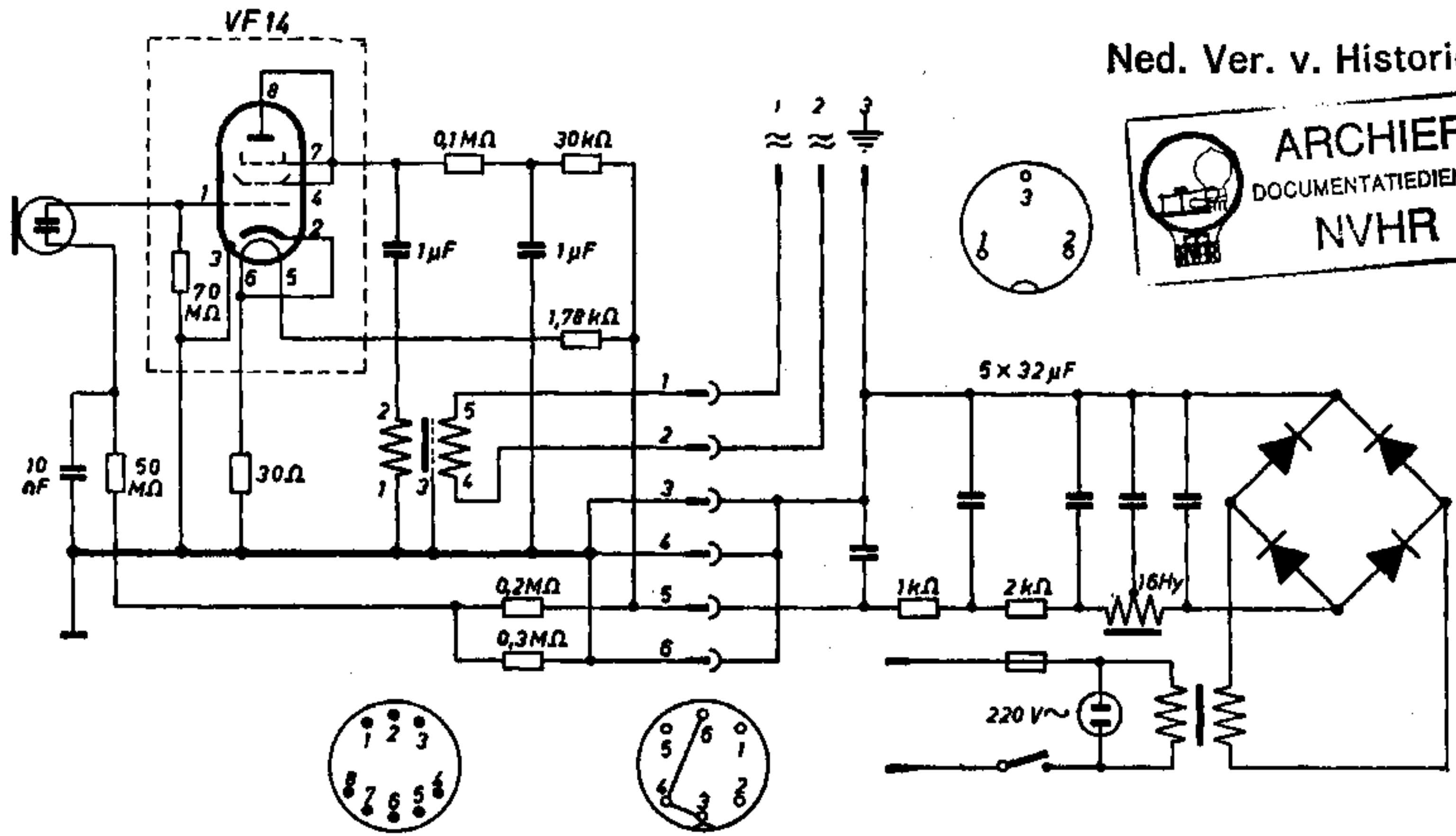
Sockelschaltung
