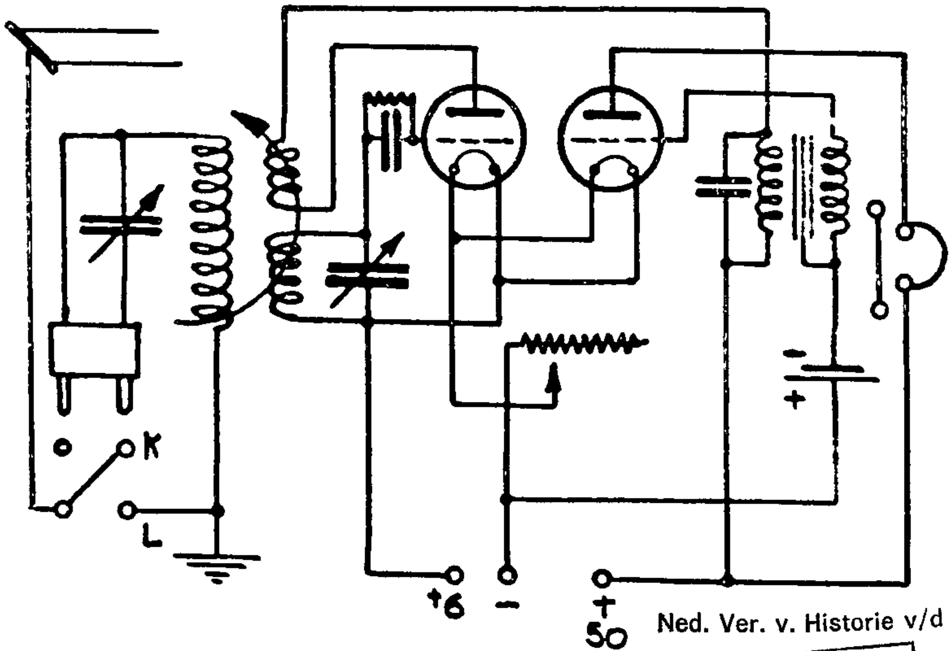
Schakelschema van ontvangtoestel W3 (O47).
