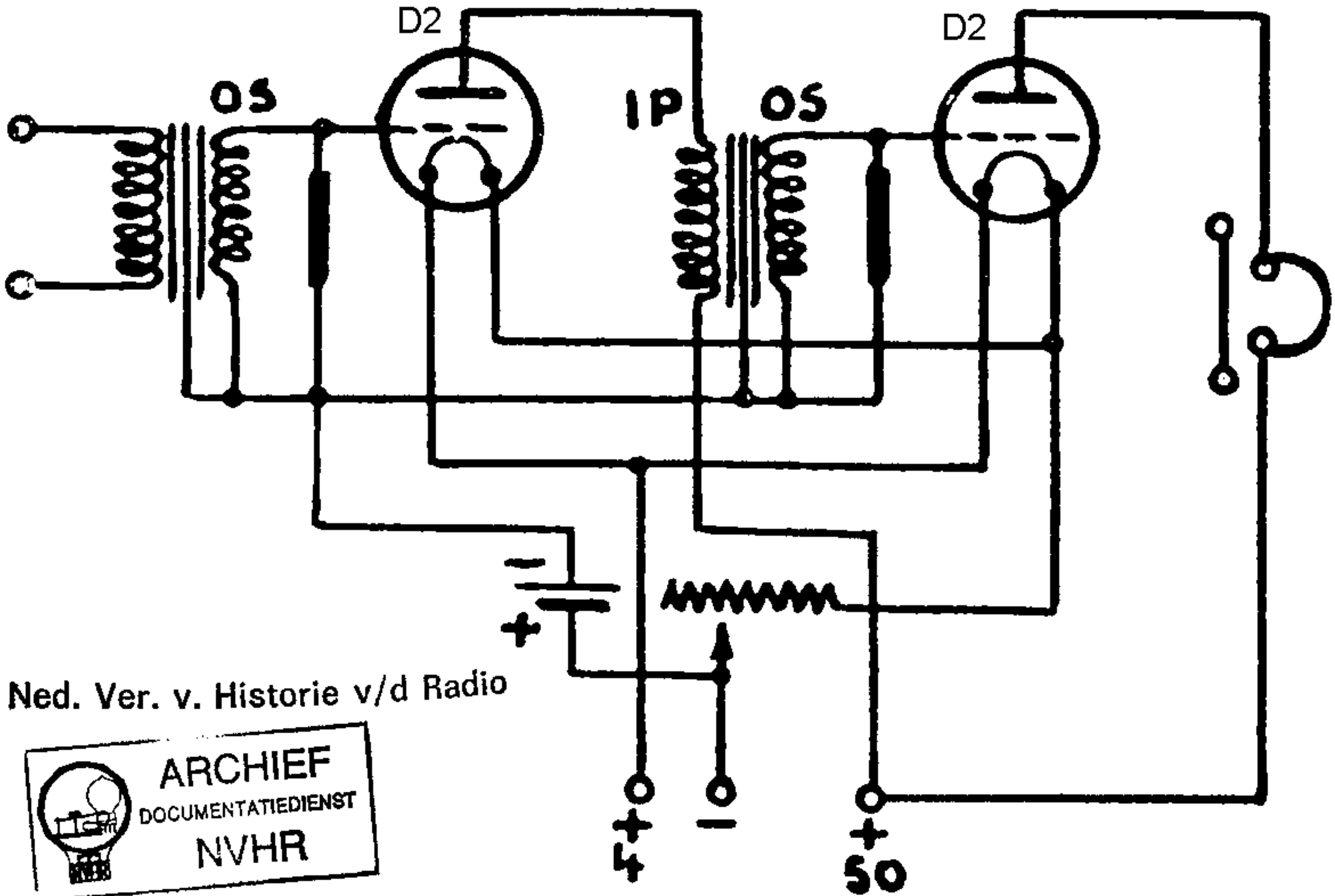
Schakelschema van versterker V3 (O42) voor Radiovox I en II.
