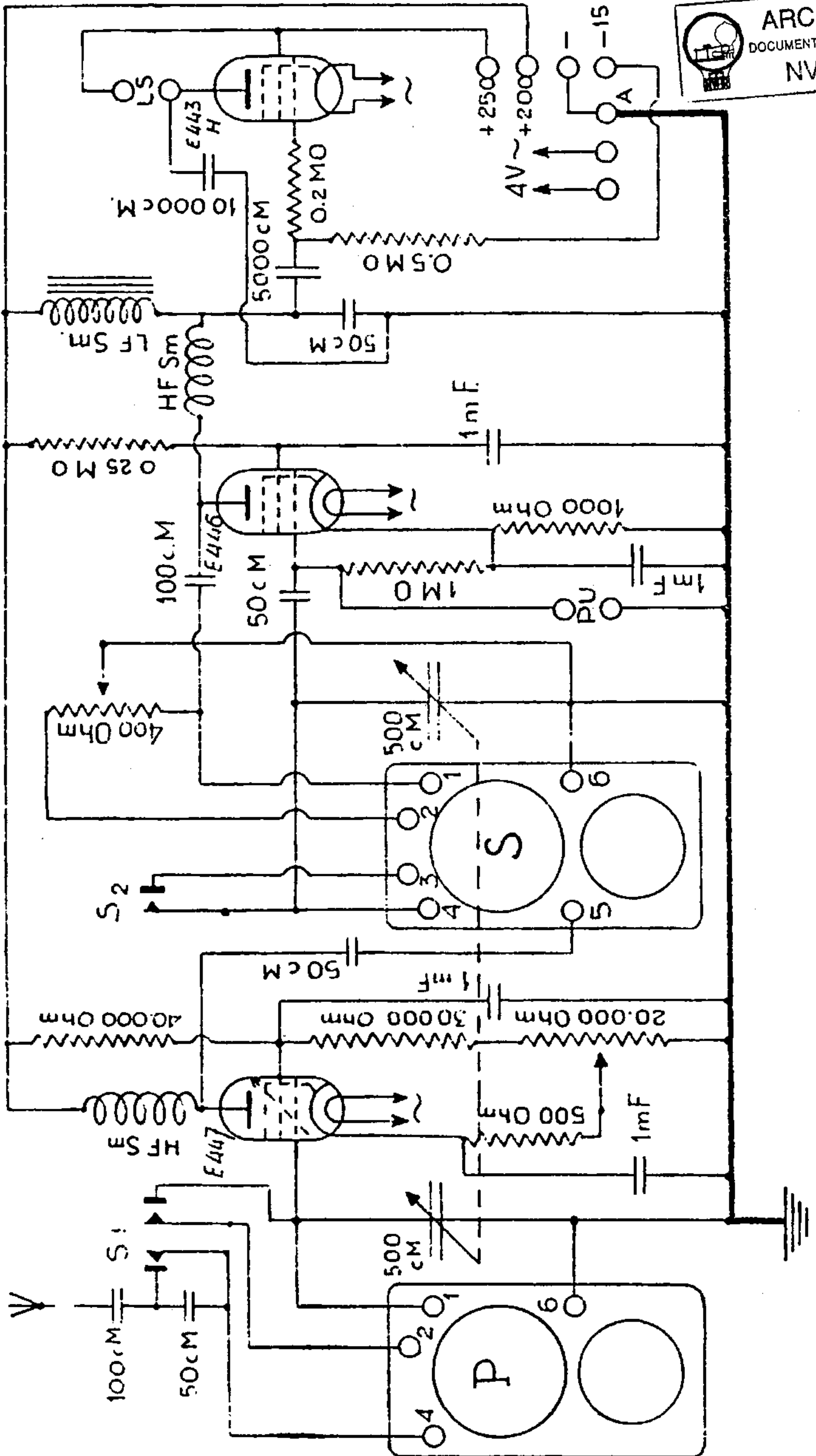
Het principe-schema.
