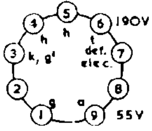
EM84 V4
