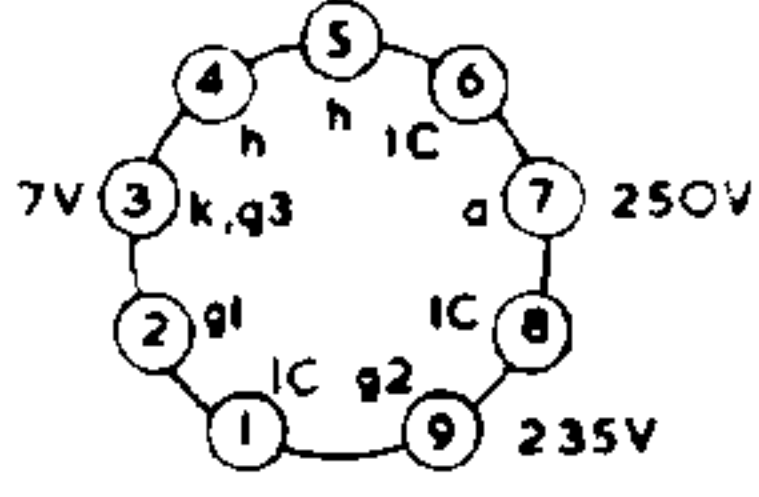
EL84 V5
