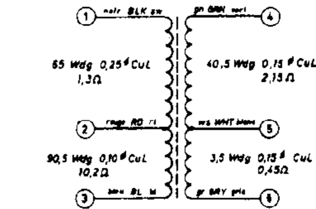
BV 9281—220 (TK 19 L)
