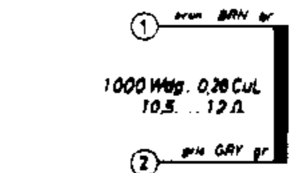
Saugkreisspule ABSORPTION COIL Bobine d'absorption BV 9230—001 (TK 14, 17, 27 L)
