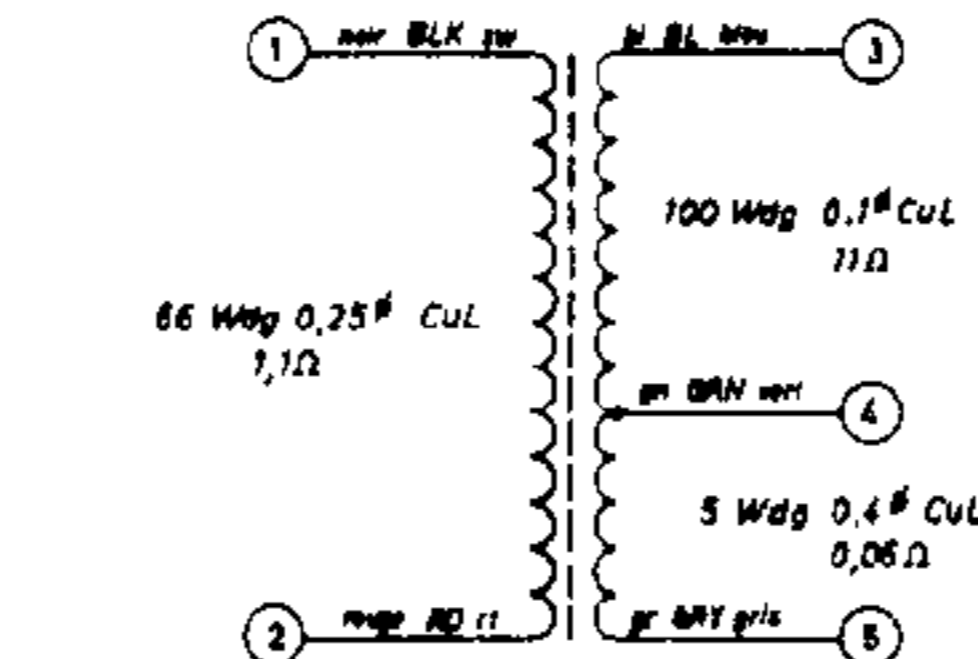
BV 9281—211 (TK 27 L)
