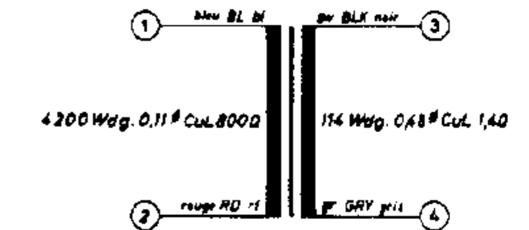
Ausgangstrafo OUTPUT TRANSFORMER Transfo de sortie BV 9054—509 (TK 14, 17, 19, 23 L)
