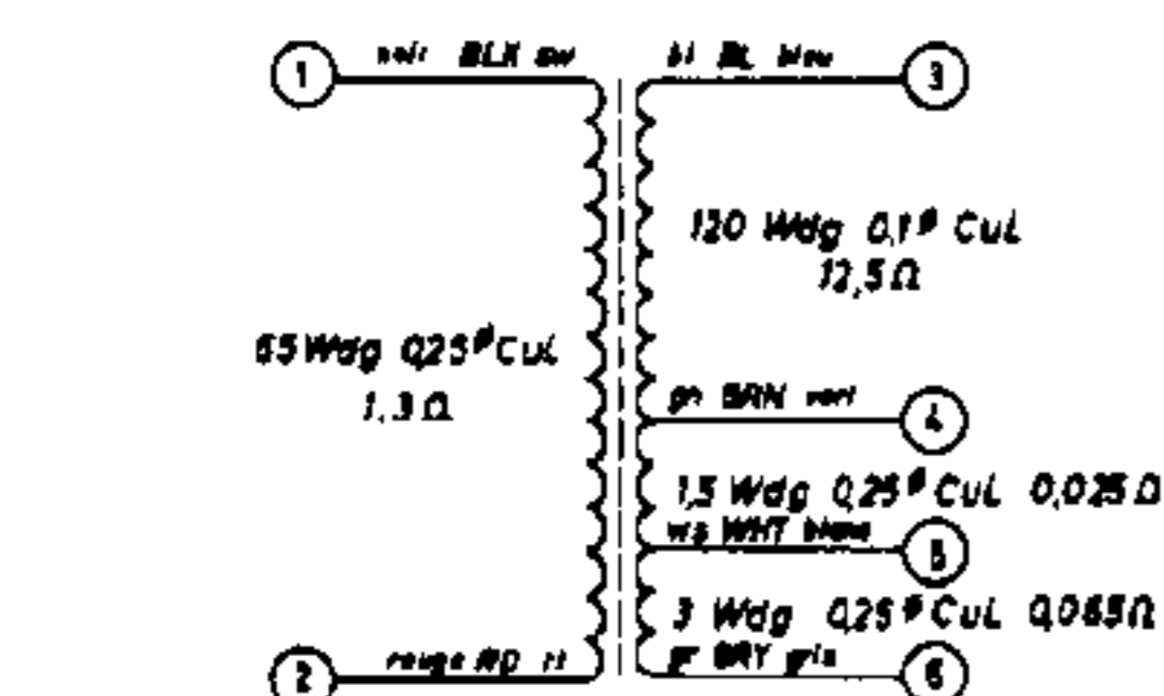
BV 9281—097 (TK 23 L)
