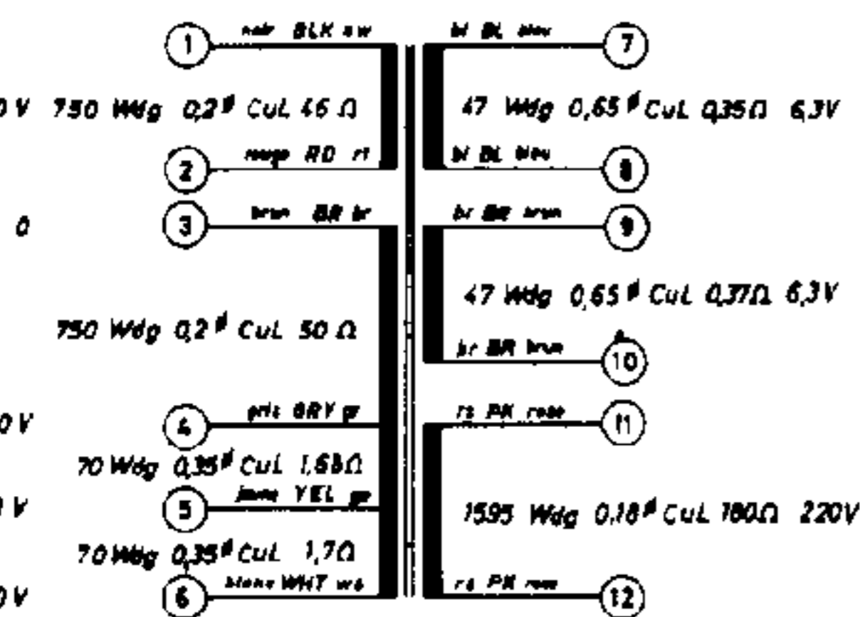
BV 9005—537 (TK 27 L)
