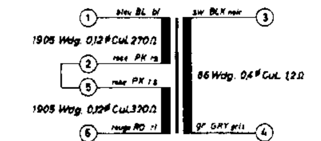
BV 9054—508 (TK 27 L)
