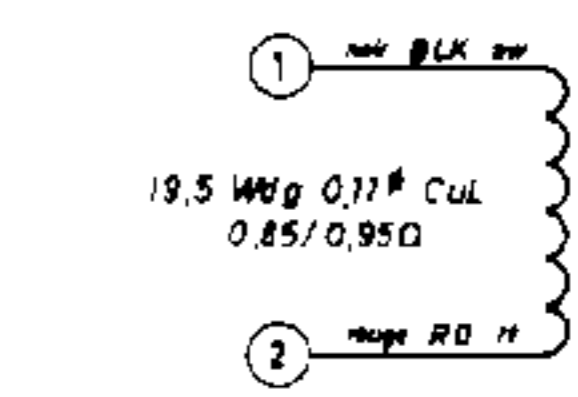
HF Drosselspule HF CHOKE Bobine d'absorption HF BV 9281—070 (TK 27 L)
