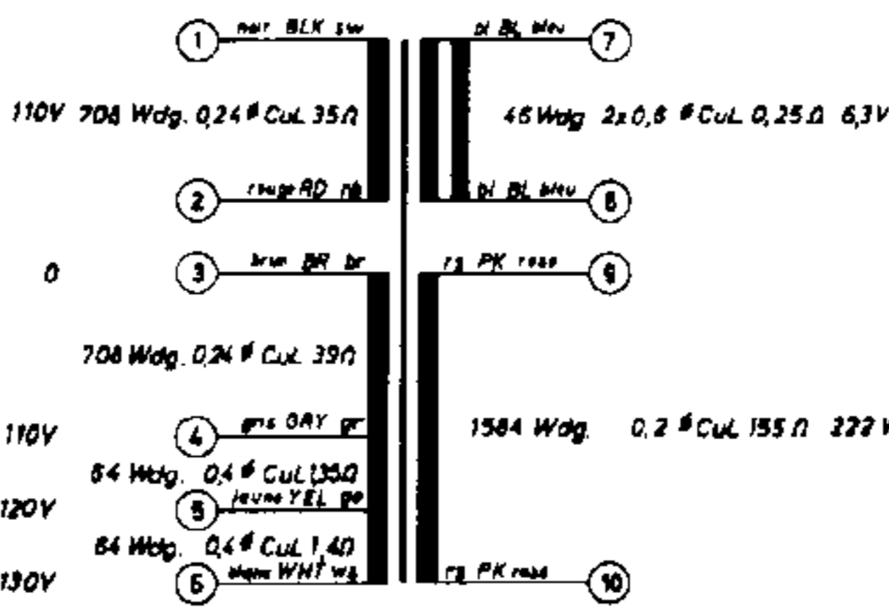
BV 9005—542 (TK 23 L)
