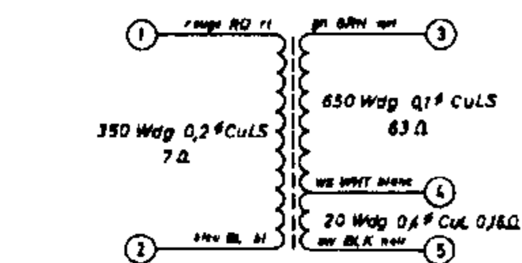
BV 9281—225 (TK 17 L)
