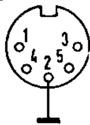
Kontakte an der Anschlußbuchse nach DIN 41524
