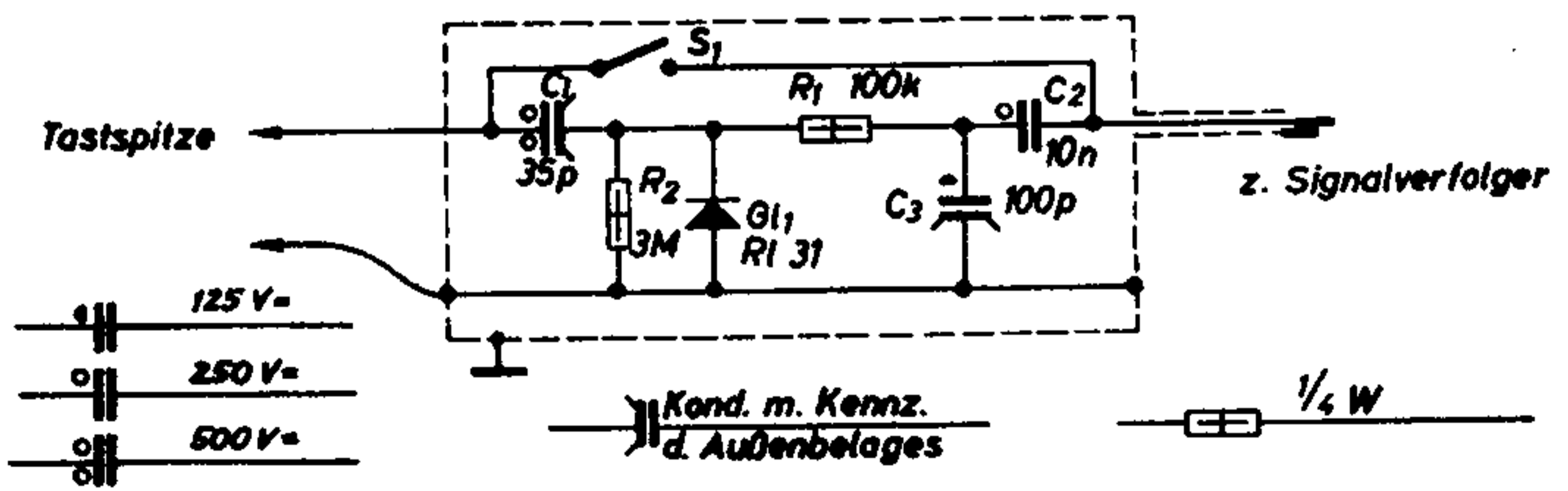
„ Tastkopf UK 1 ” (6057-001)
