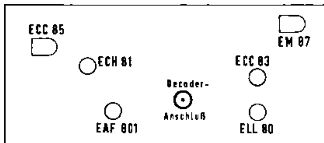
Chassis von oben gesehen (Röhrenlageplan)
