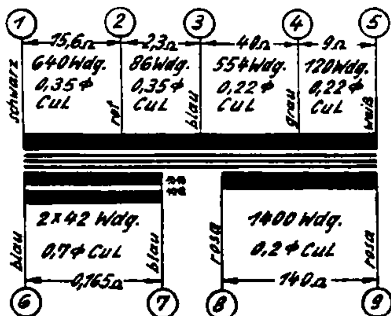
Netztransformator BV 78/33
