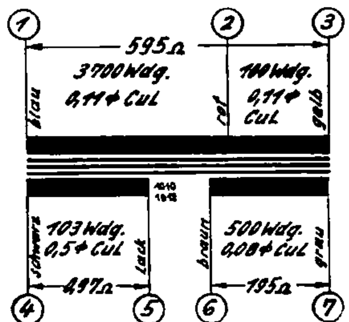
Übertrager 48/26
