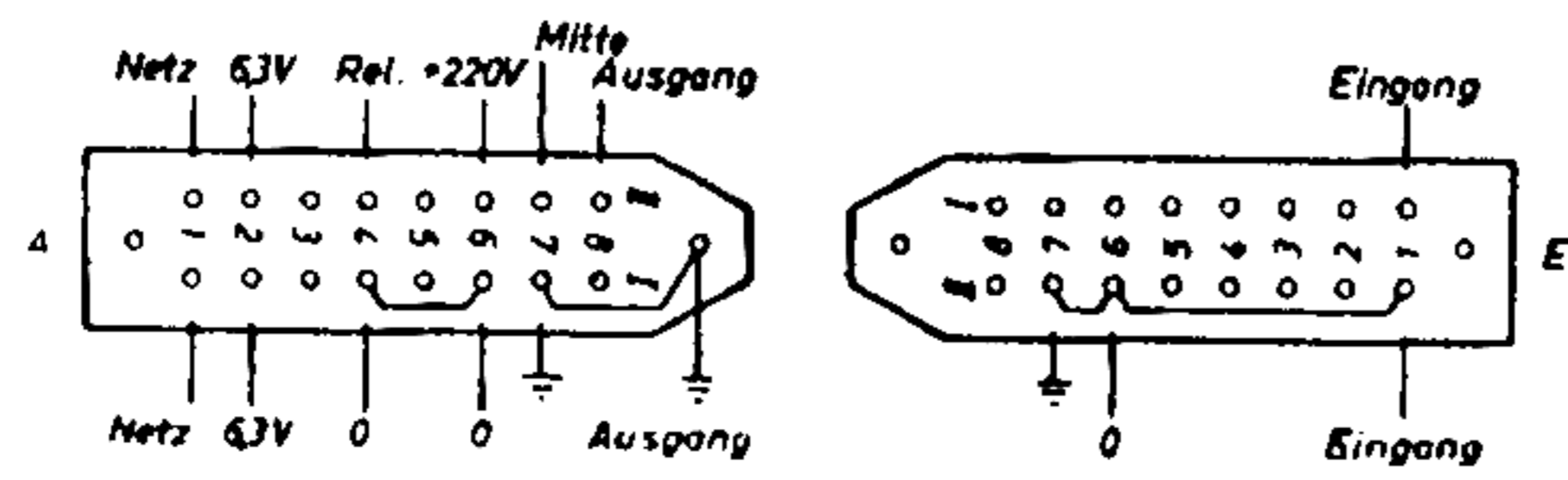
Steckerteisten von hinten gesehen
