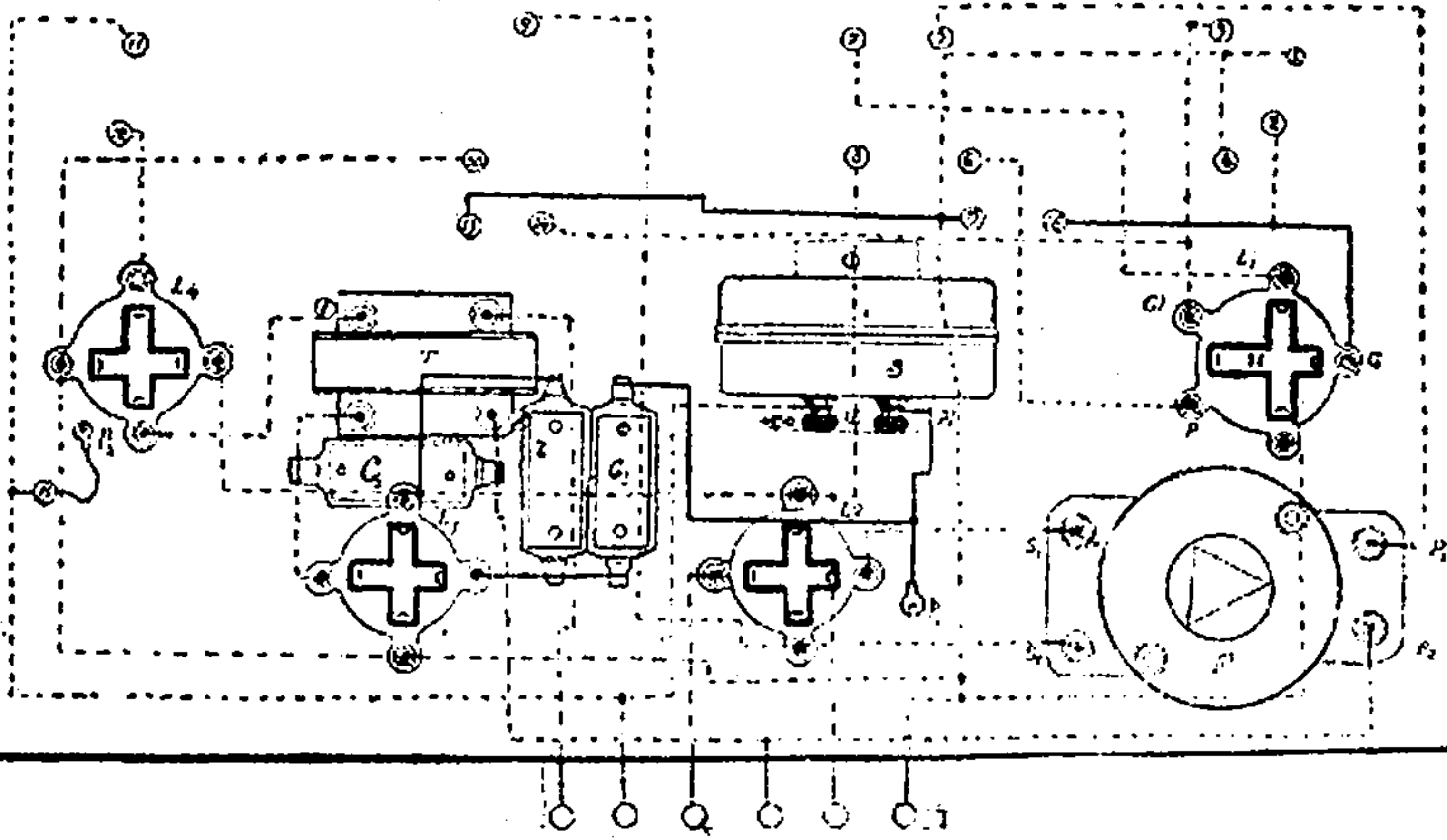
Fig. 203.—Supradyna FAR, cu patru lămpi, schema de conexiuni.
