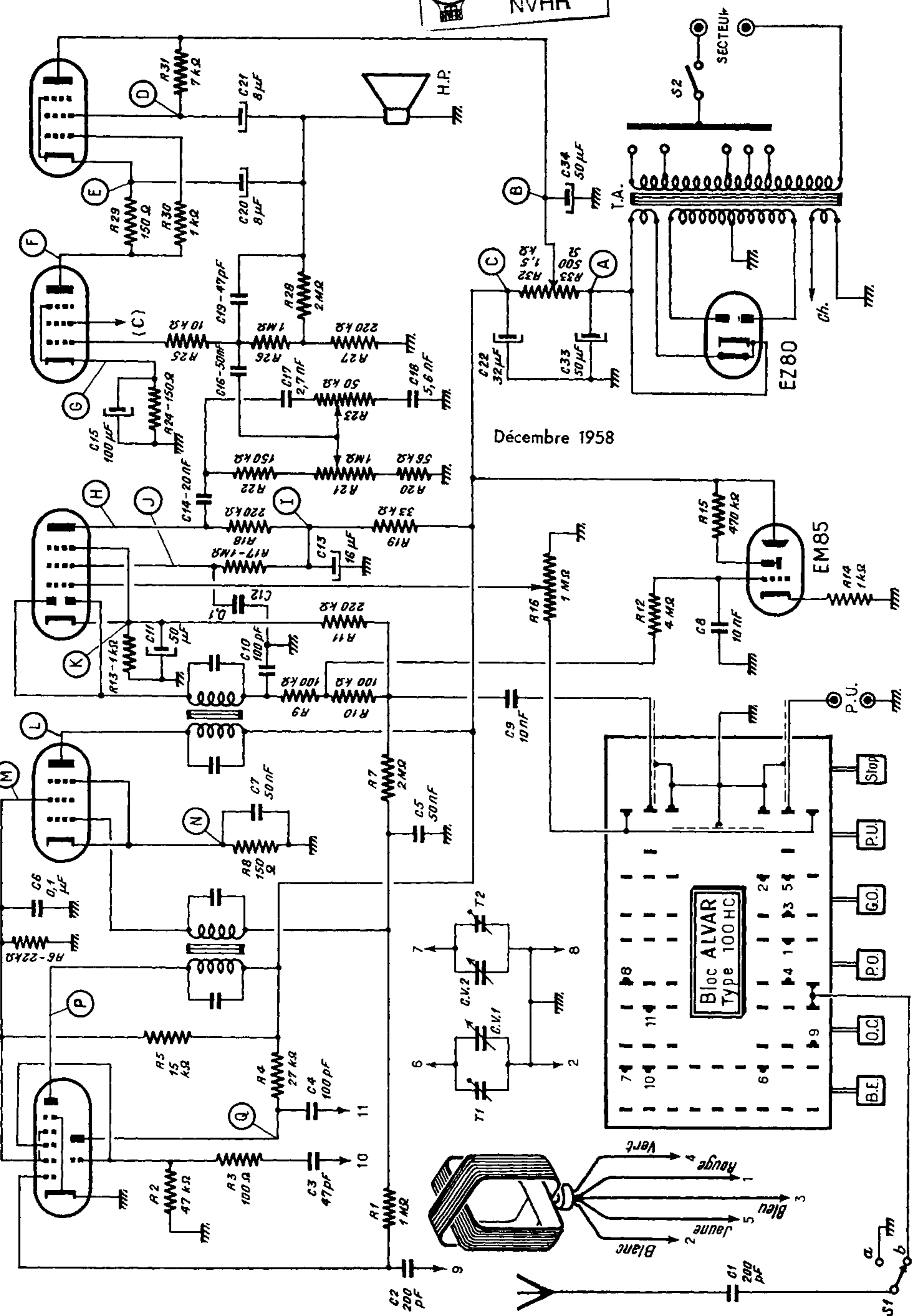
Schéma général du récepteur "Caravelle" et le branchement du bloc de bobinages
