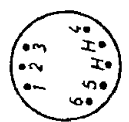
ECF12, EF12, EL13 Sockettschaltungen
