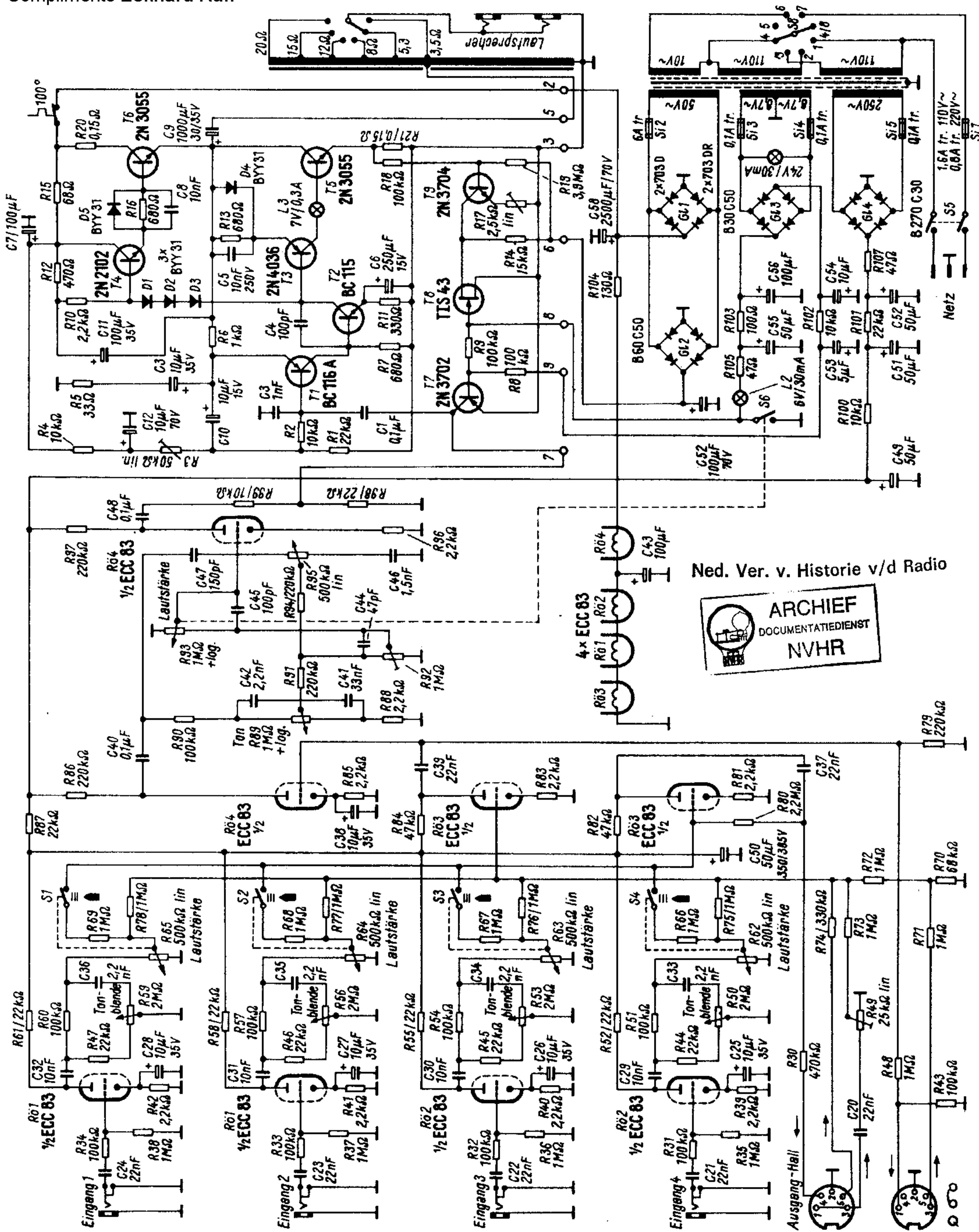
Bild 11. Schaltbild des Gesangverstärkers M 100 (Kliment-Echolette)
