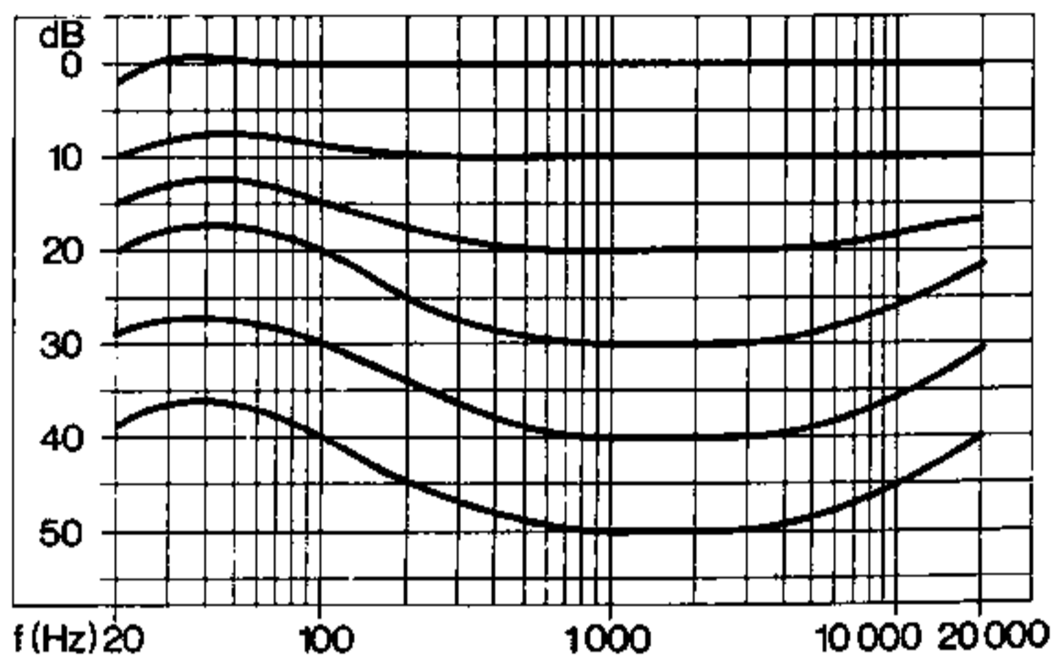
Fig. 4 Wirkungsweise der physiologischen Lautstärkeregelung. 0 dB = Lautstärkeregl. offen
