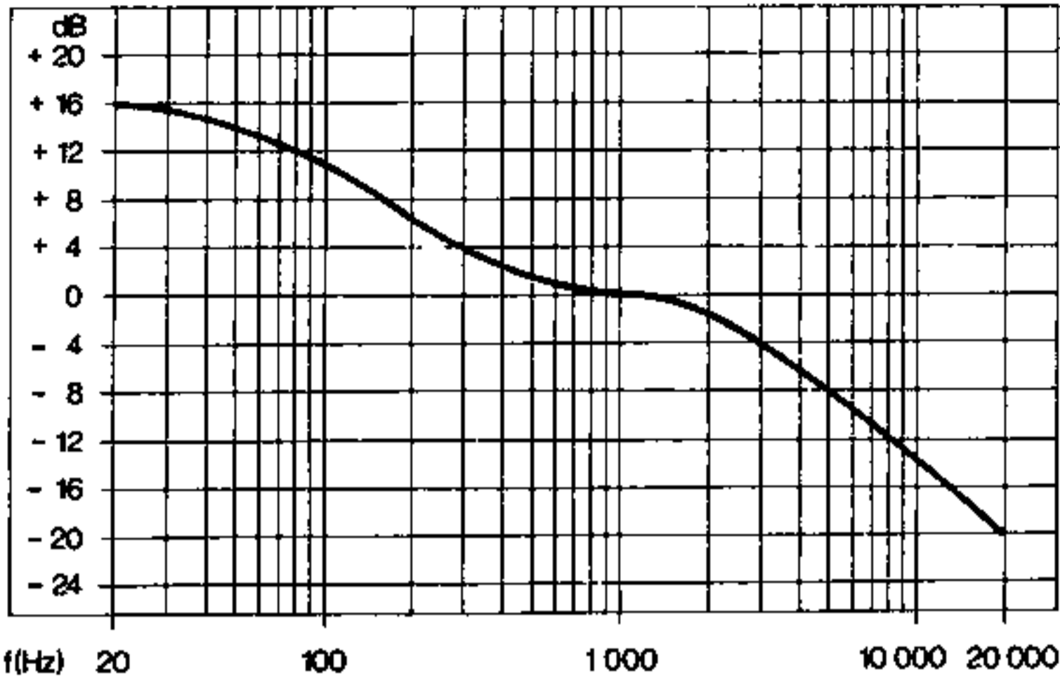
Fig. 3 Wirkungsbereiche der Klangregler. 0 dB = Bass- und Höhenregler in Mittenstellung
