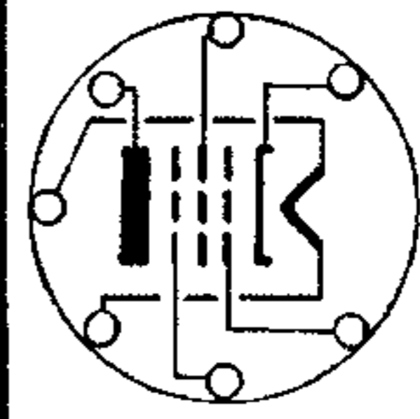
12BA6
