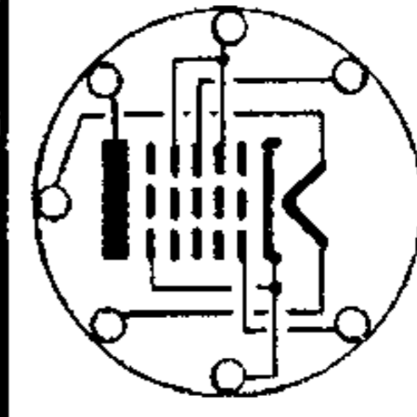
12BE6
