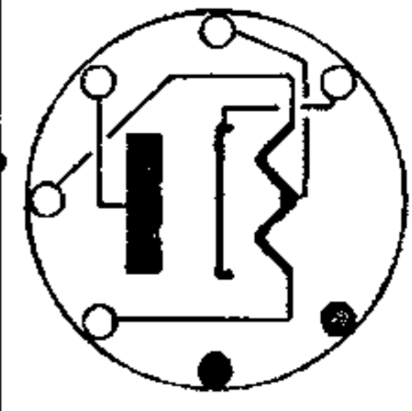
35W4
