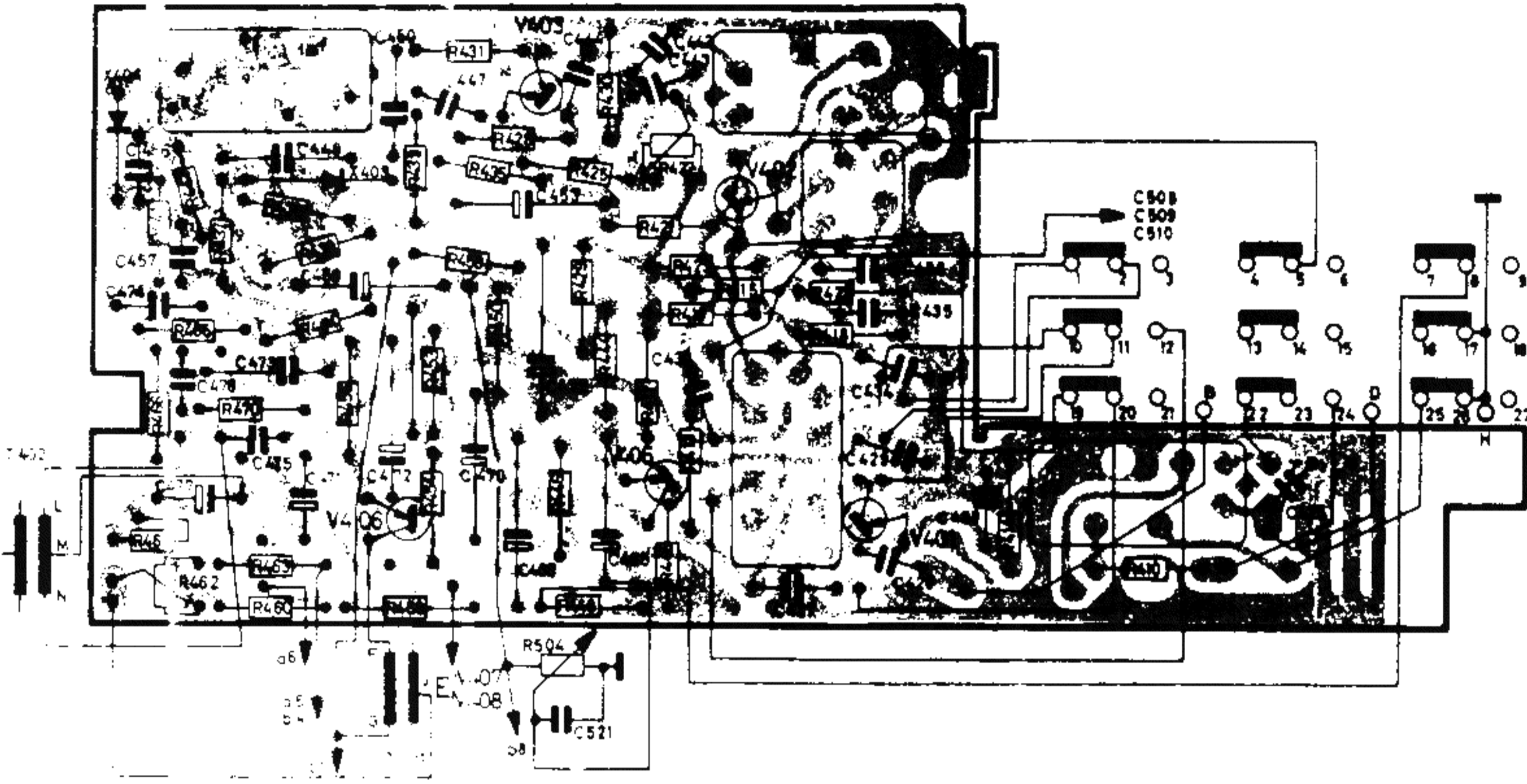
Fig. 26 Bestückungsseite Components side
