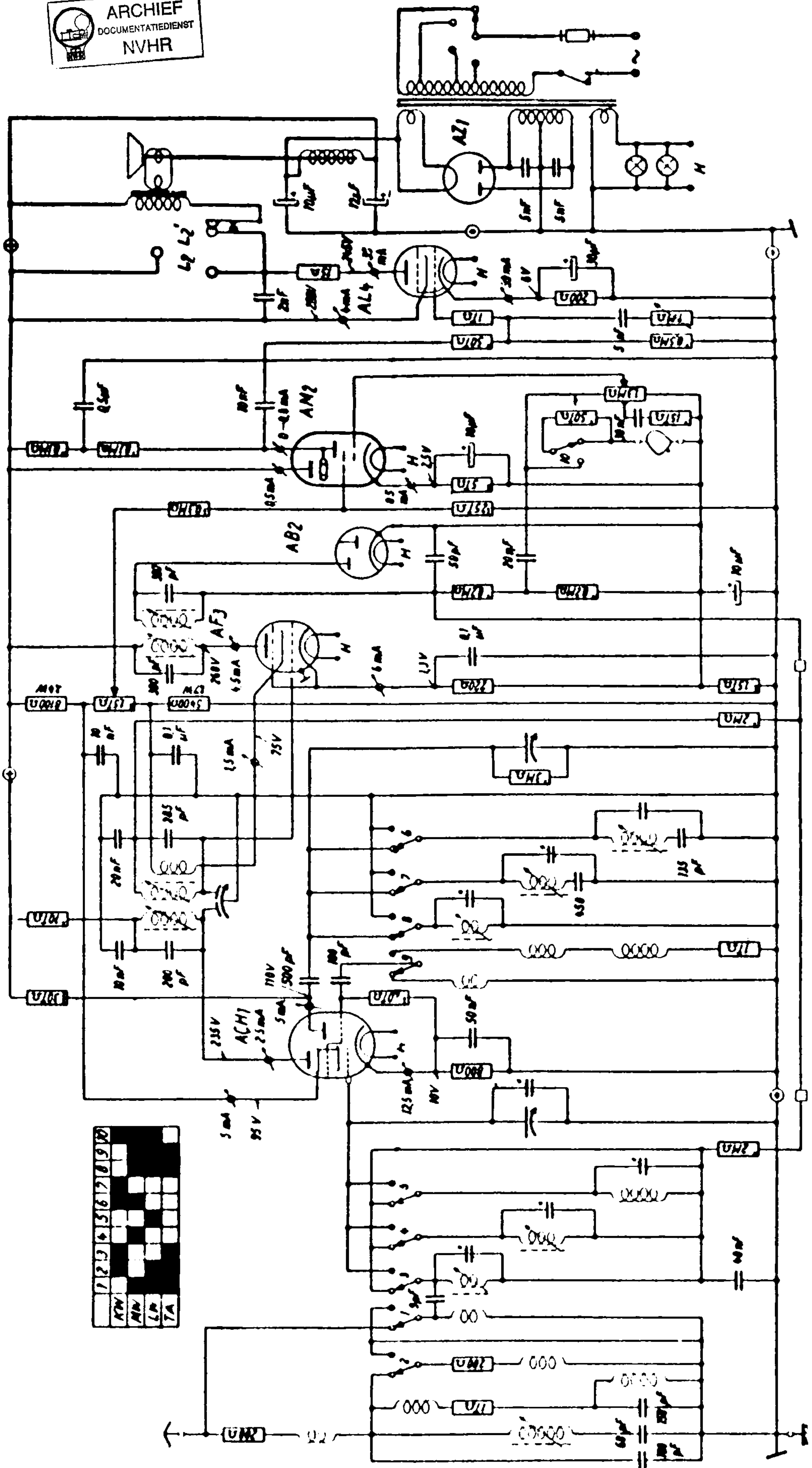
Ideal, 4W 77 und Hagenuk, 648 KW, Wechselstrom, 1 Vorkreis, 4 Zwischenfrequenzkreise
