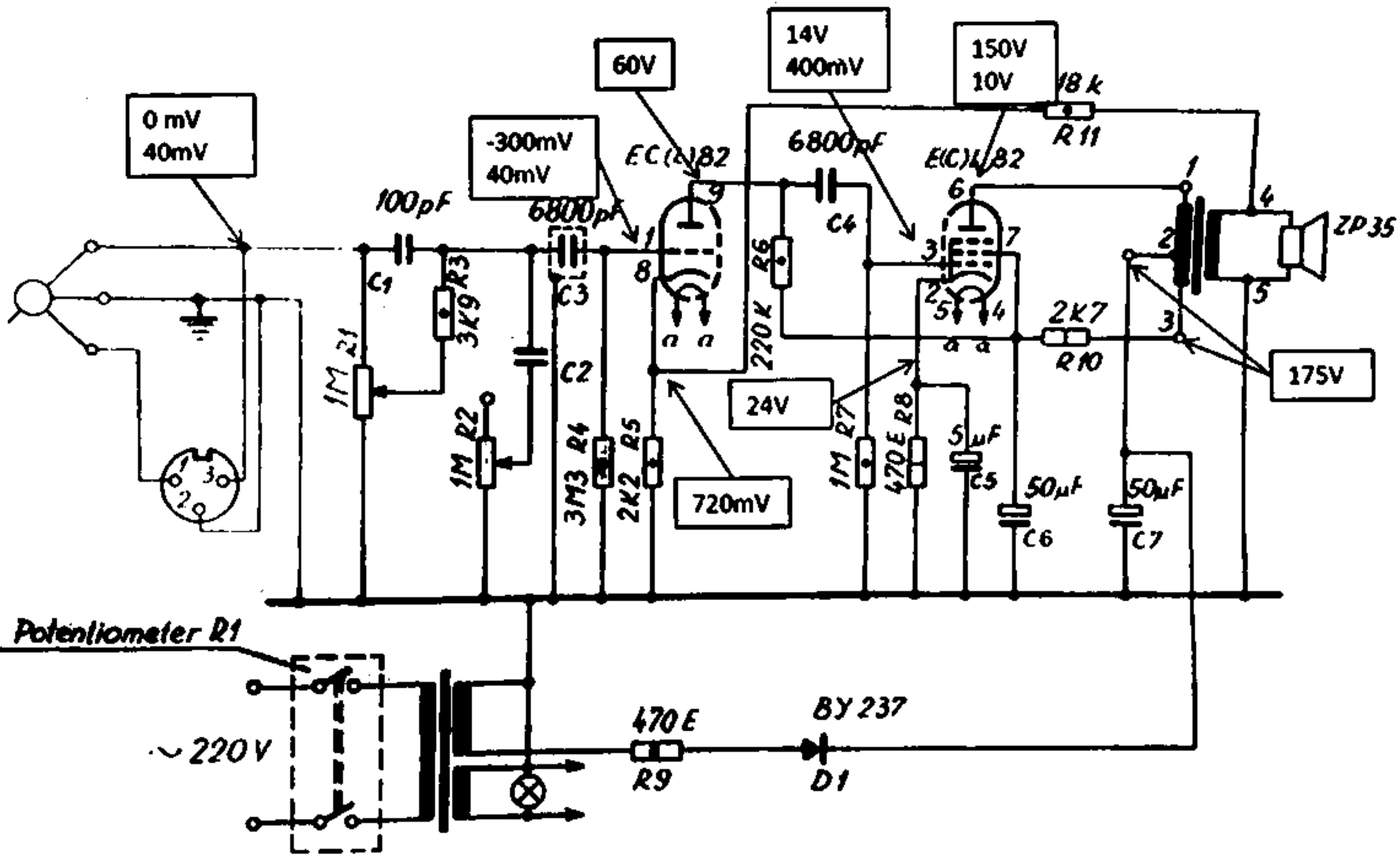
Schaltbild zum Plattenspielerkoffer Stockholm Studio 90
