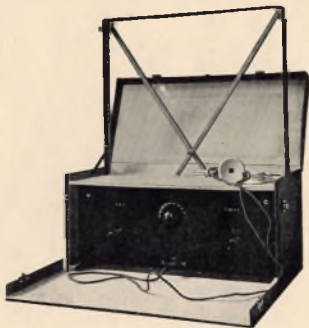
ONTVANGTOESTEL N. R. W. KAMPEERMODEL IN KOFFER.
