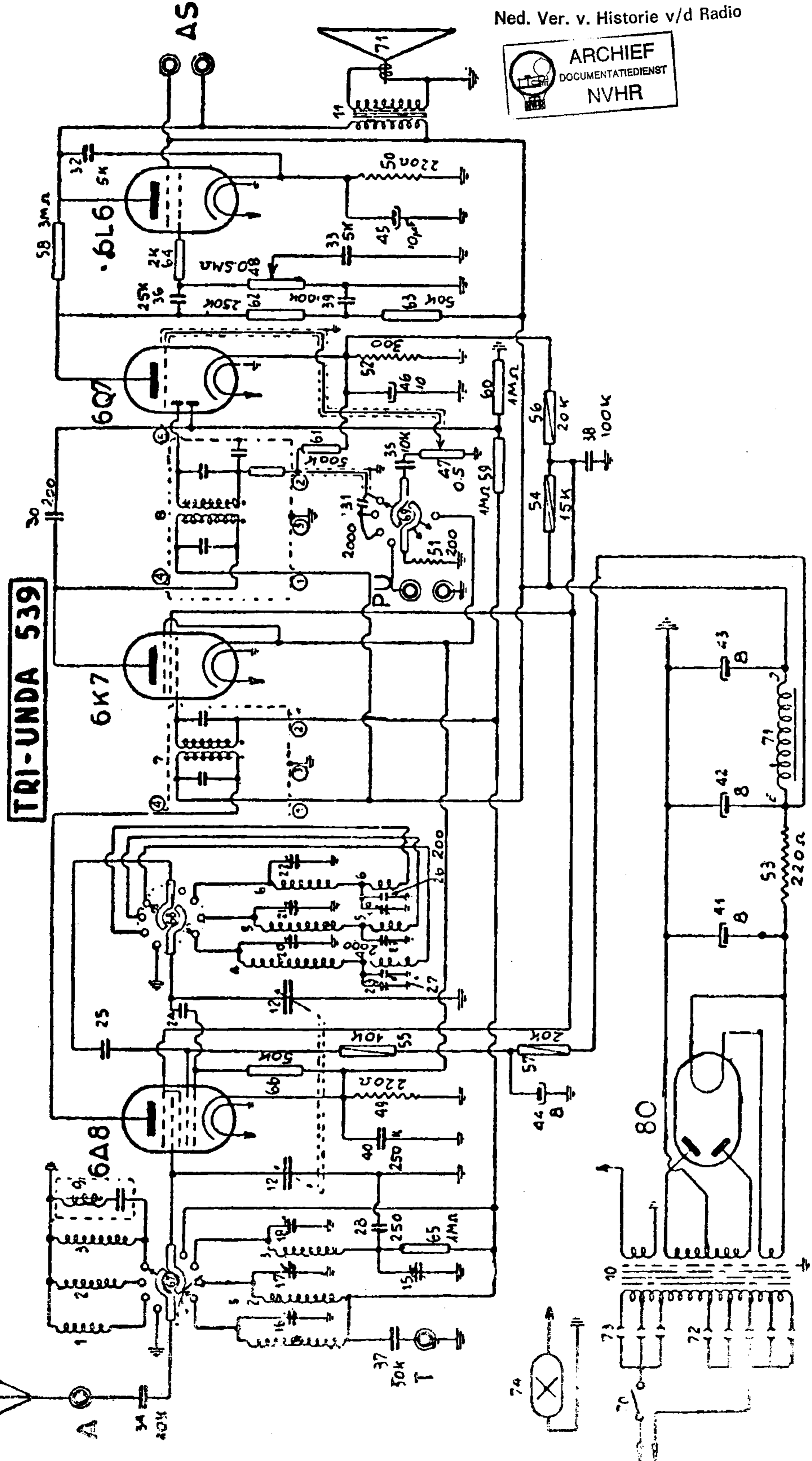
UNDA RADIO. — Modello Tri-Unda 539. — Produzione 1938-39. — Gàmme: cc. (15-30), c. (30-80), m. (206,5-600). — Potenza d'uscita: 5,5 W. — Media frequenza: 450 kHz.
