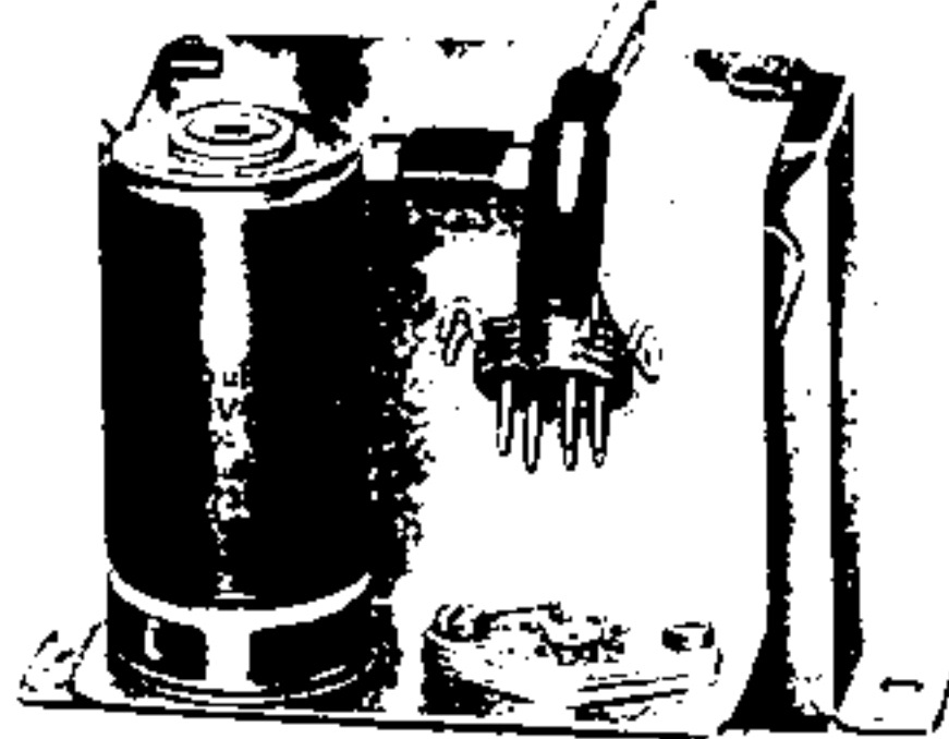
Telaio di alimentazione. Le dimensioni del sintonizzatore sono 175 x 130 x 98 mm, quelle dell'alimentatore 94 x 72 x 75 mm.
