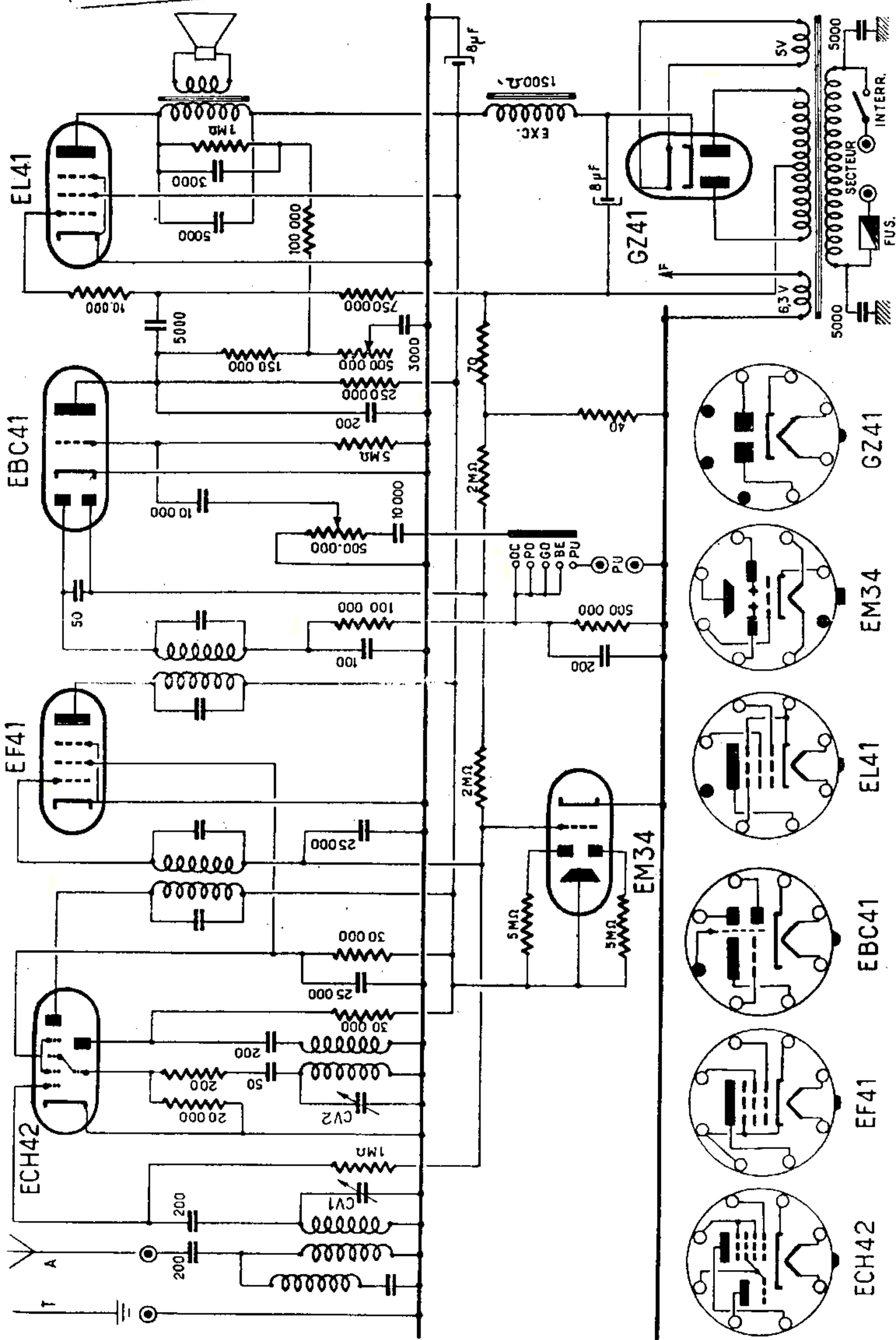
Schéma général des récepteurs « Dauphin » et « Ondine ».
