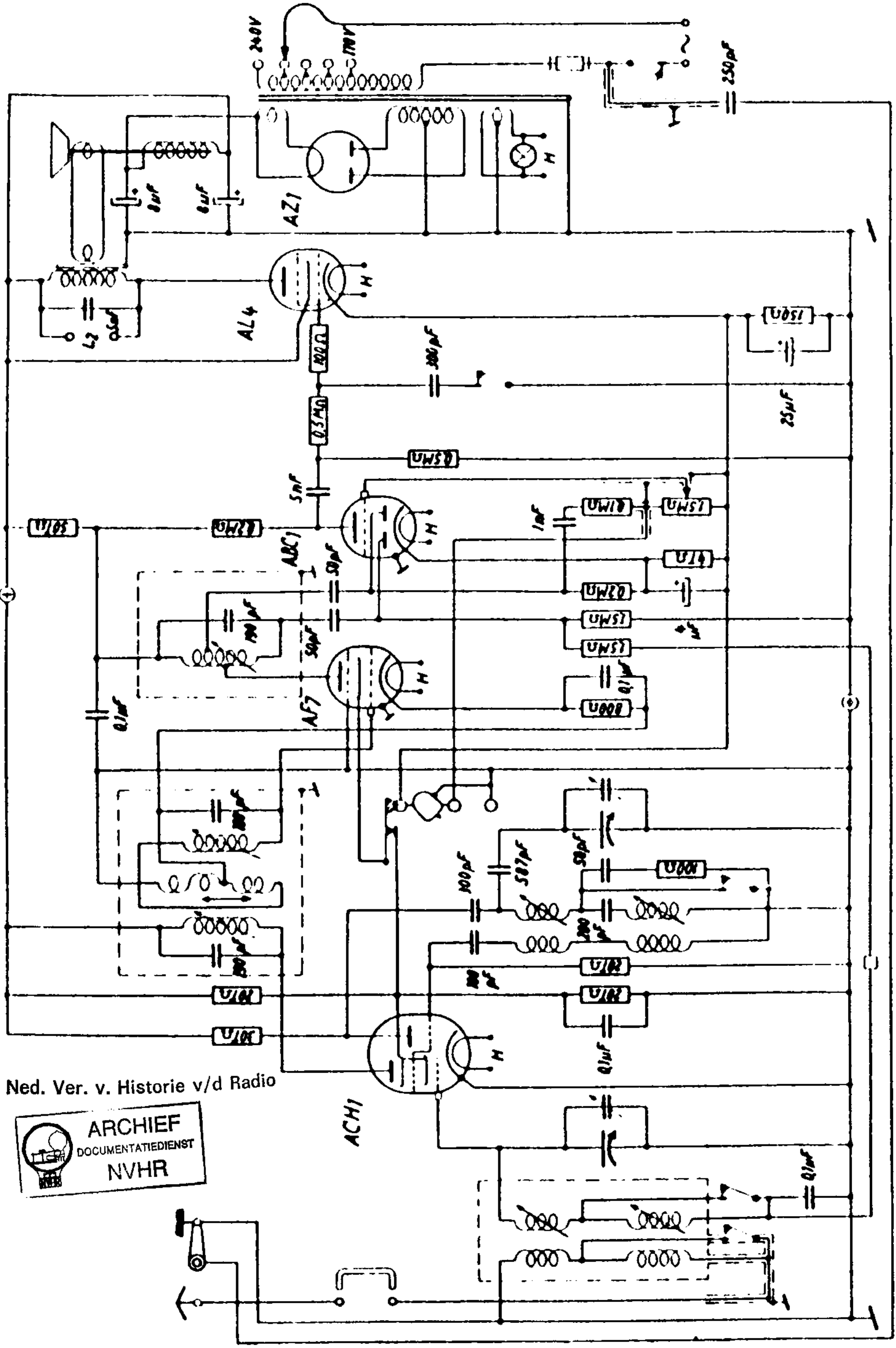
Detewe, 754W, Wechselstrom, 1 Vorkreis, 3 Zwischenfrequenzkreise
