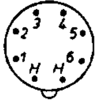
Sockelschaltung
