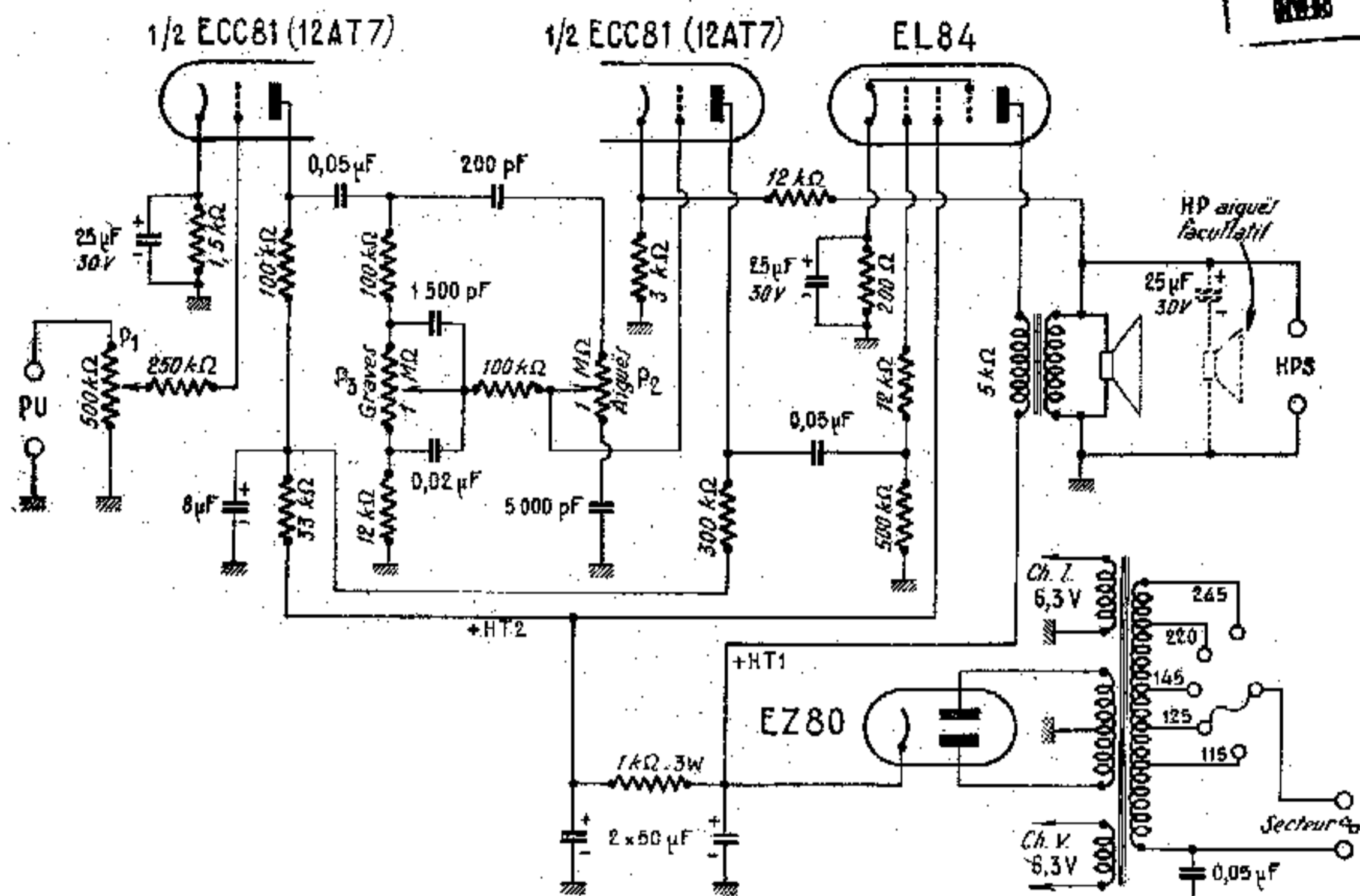
Schéma de principe de l'amplificateur
