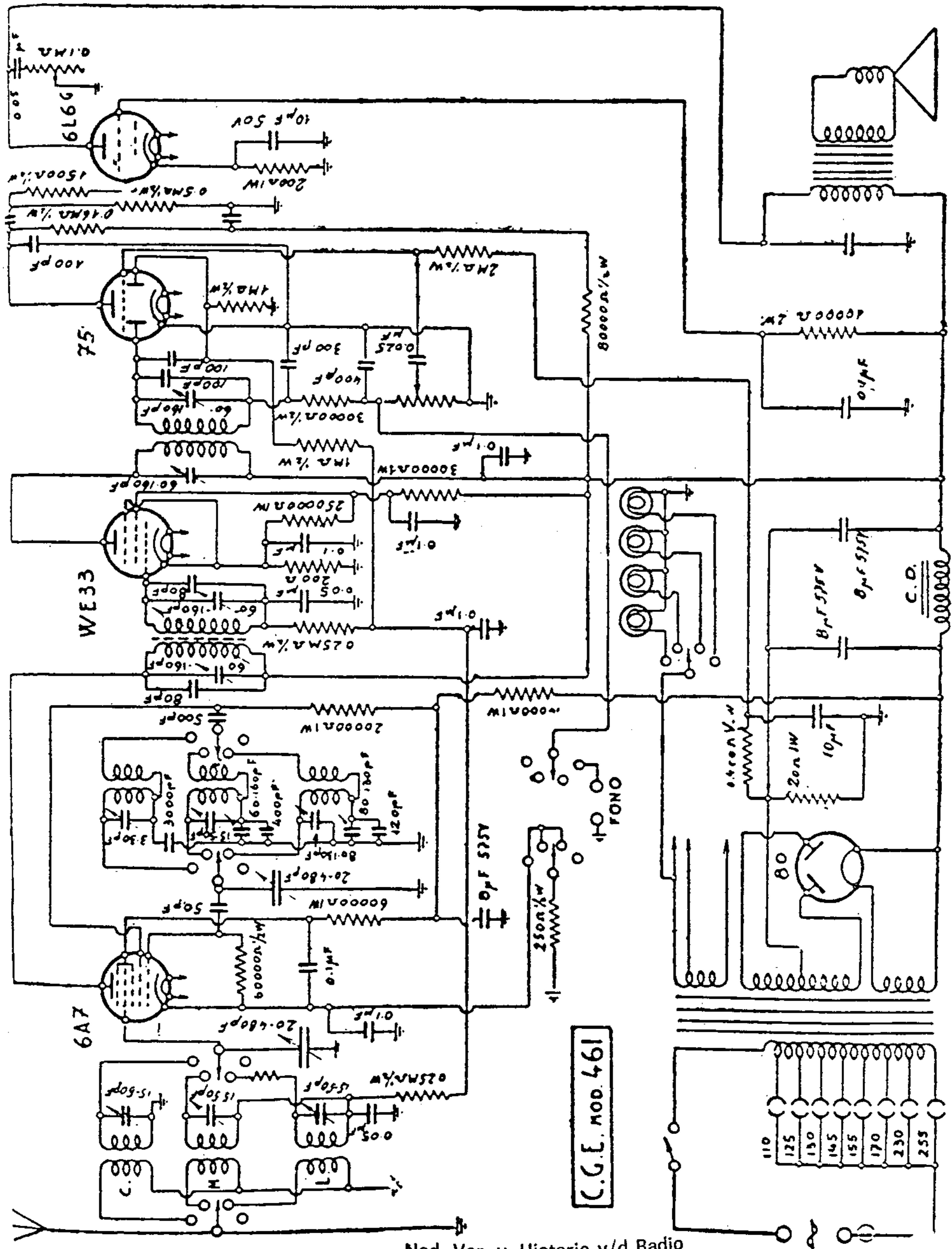
COMPAGNIA GENERALE DI ELETTRICITÀ. — Modello «461». — Produzione 1938. — Media frequenza: 459 KHZ.
