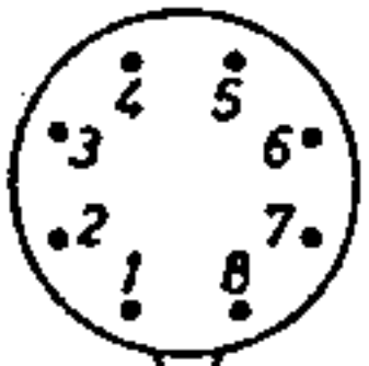
EF80 EAF42 Sockelschaltungen
