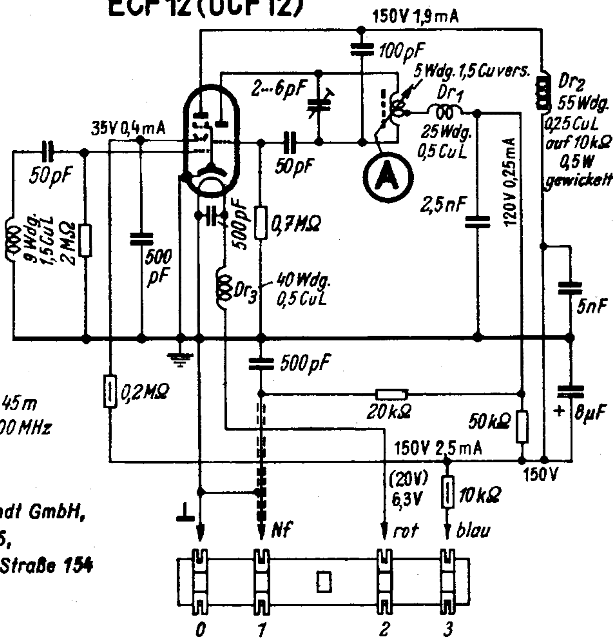
Löt-leiste Brandt-UKW-PR-E
